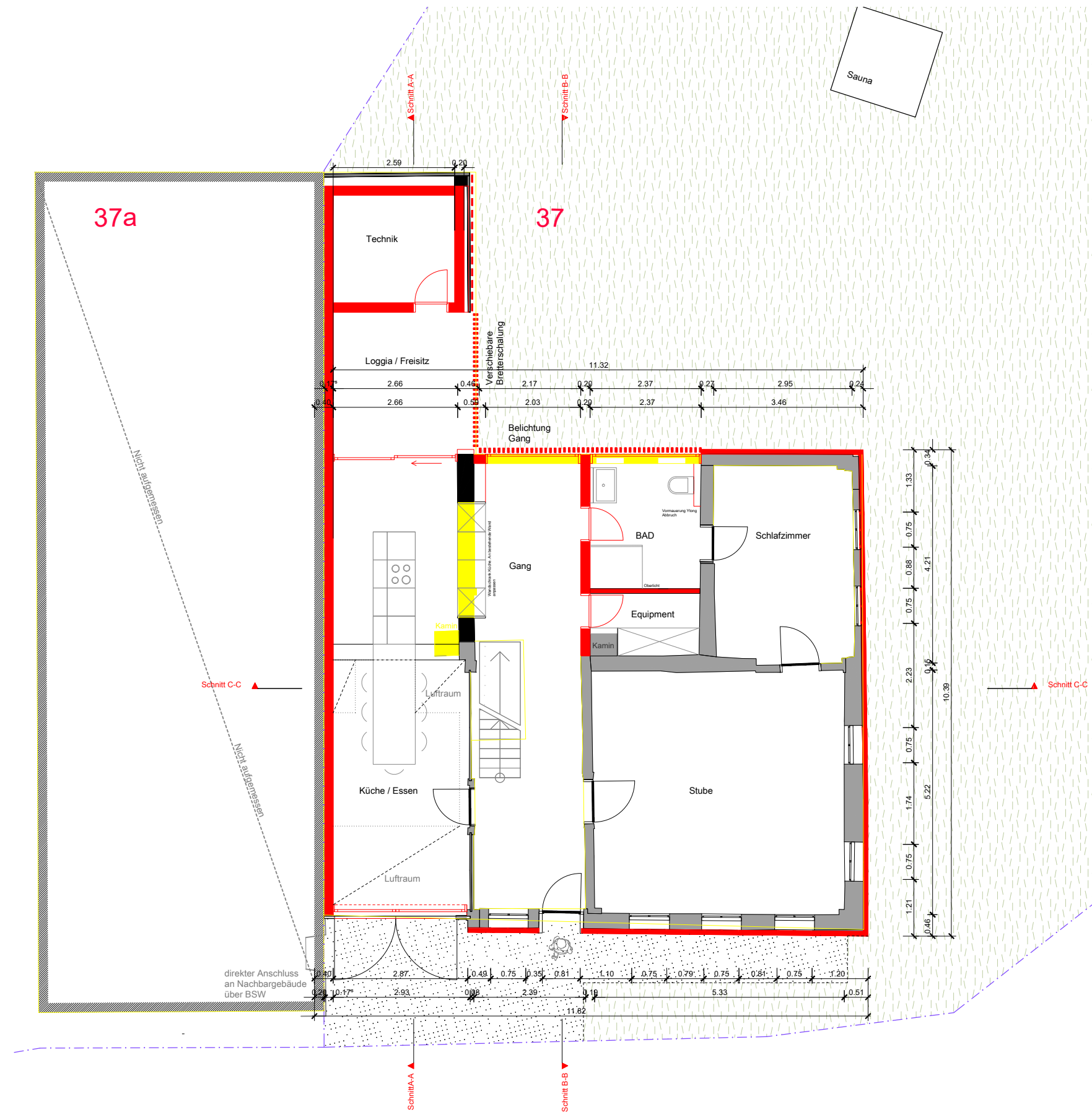
Grundriss EG
