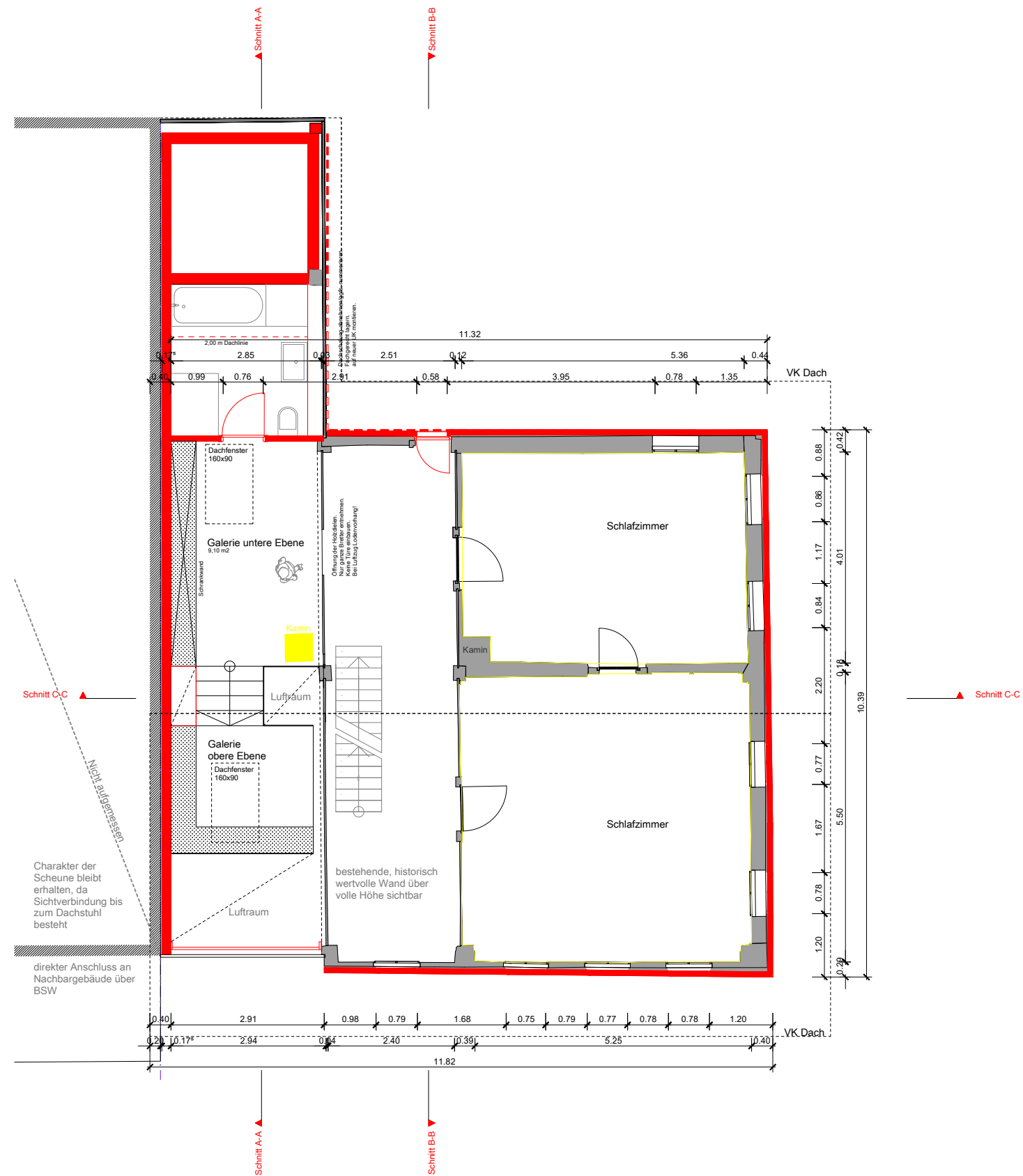
Grundriss OG
