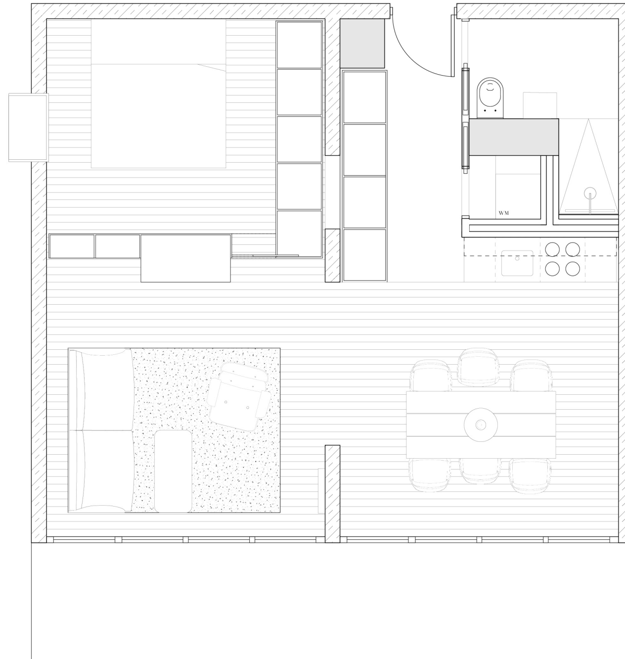
Grundriss M 1:50
