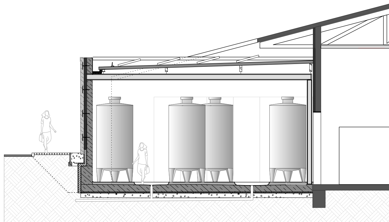
Schnitt AA
