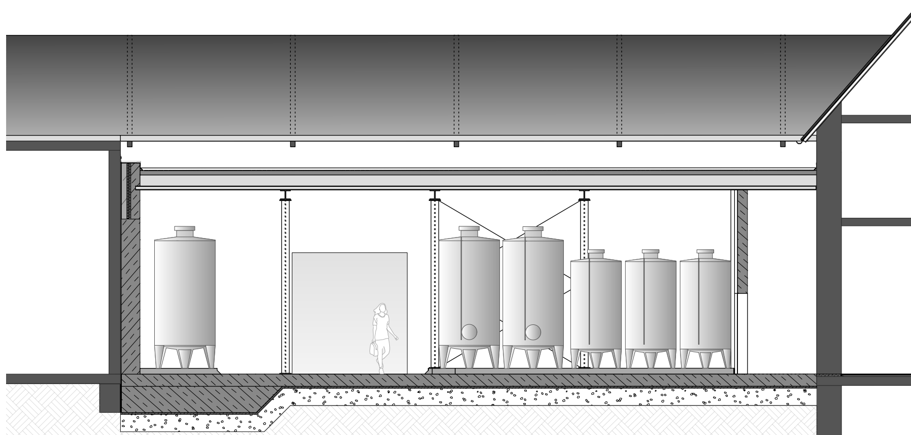
Schnitt B-B
