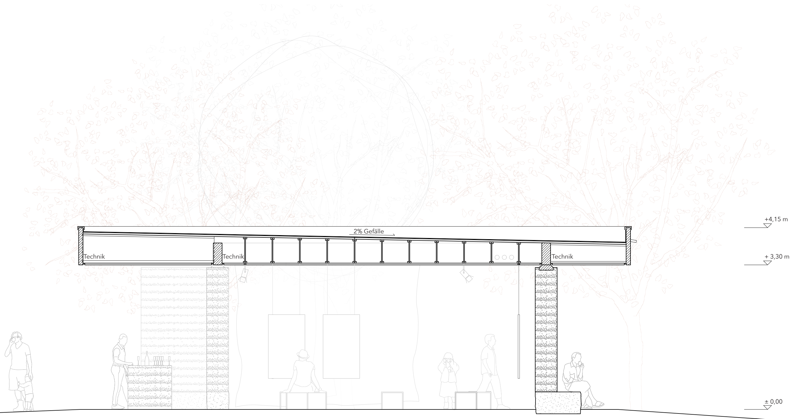
Schnitt A-A 1:50
