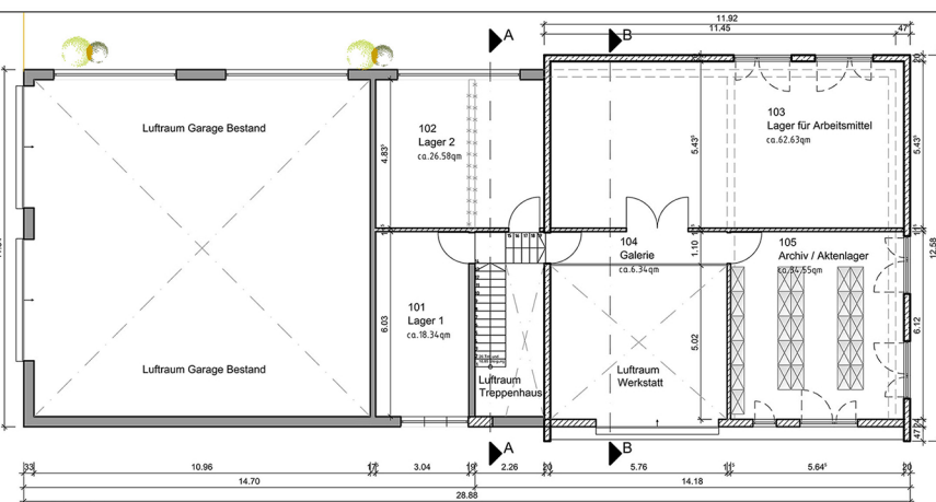
Grundriss OG
