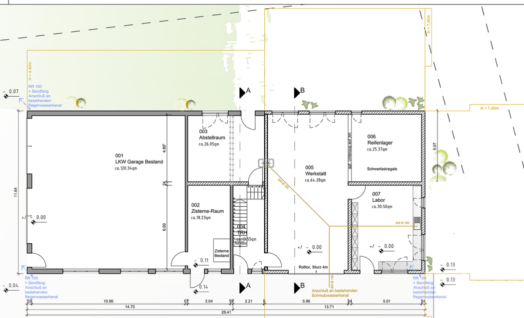
Grundriss EG mit Grundstück
