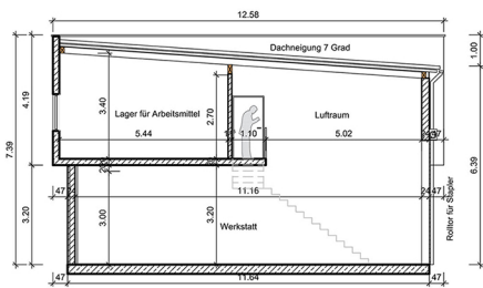
Schnitt B-B
