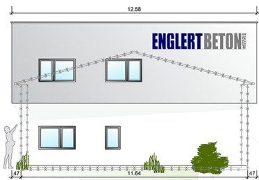
Ostansicht
