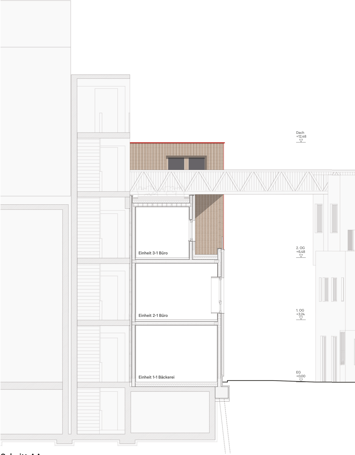
Schnitt AA
