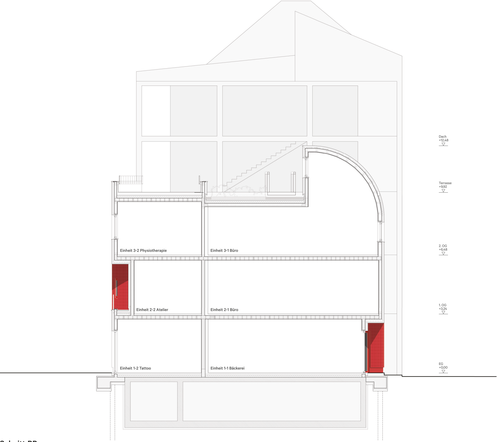
Schnitt BB
