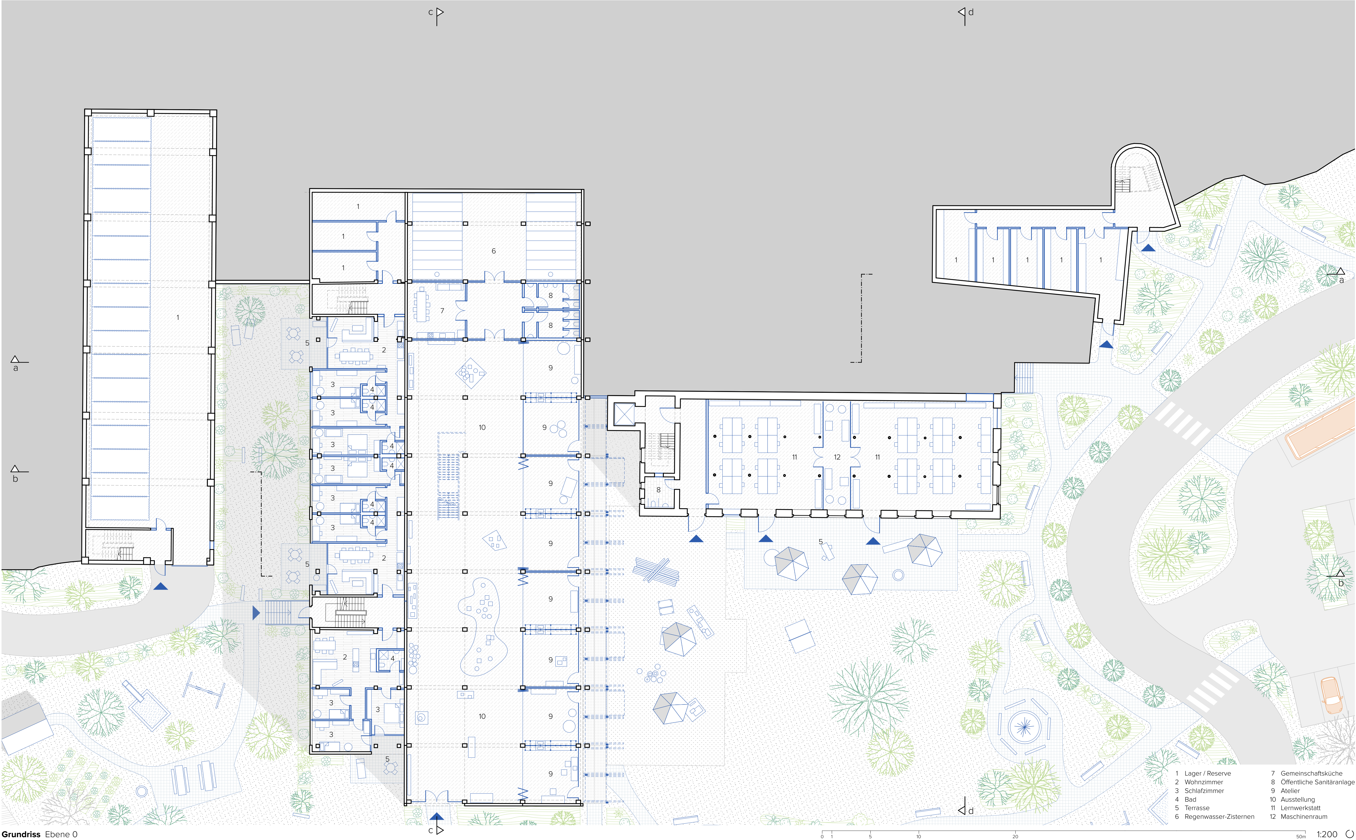
Grundriss Ebene 0
