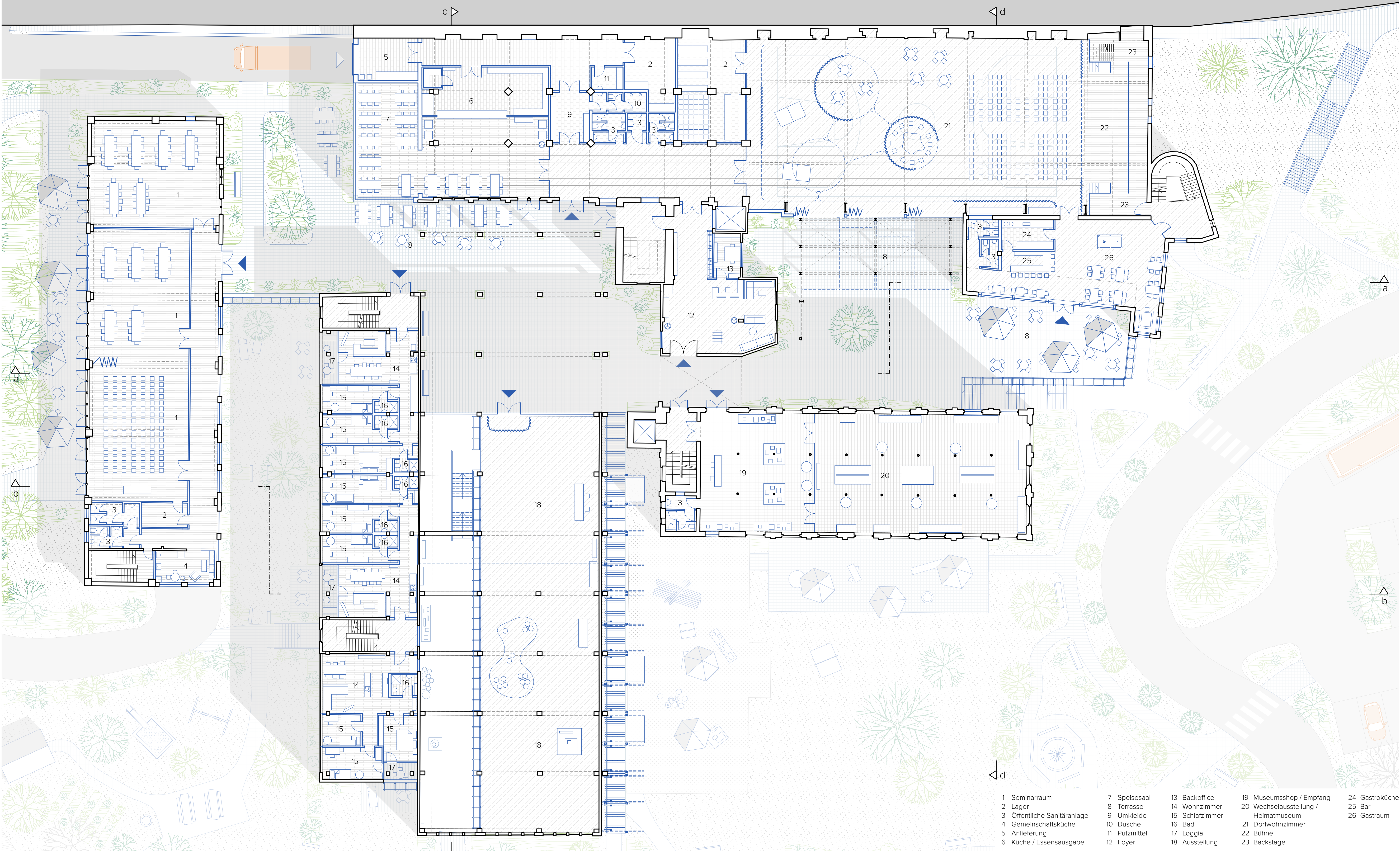
Grundriss Ebene 1
