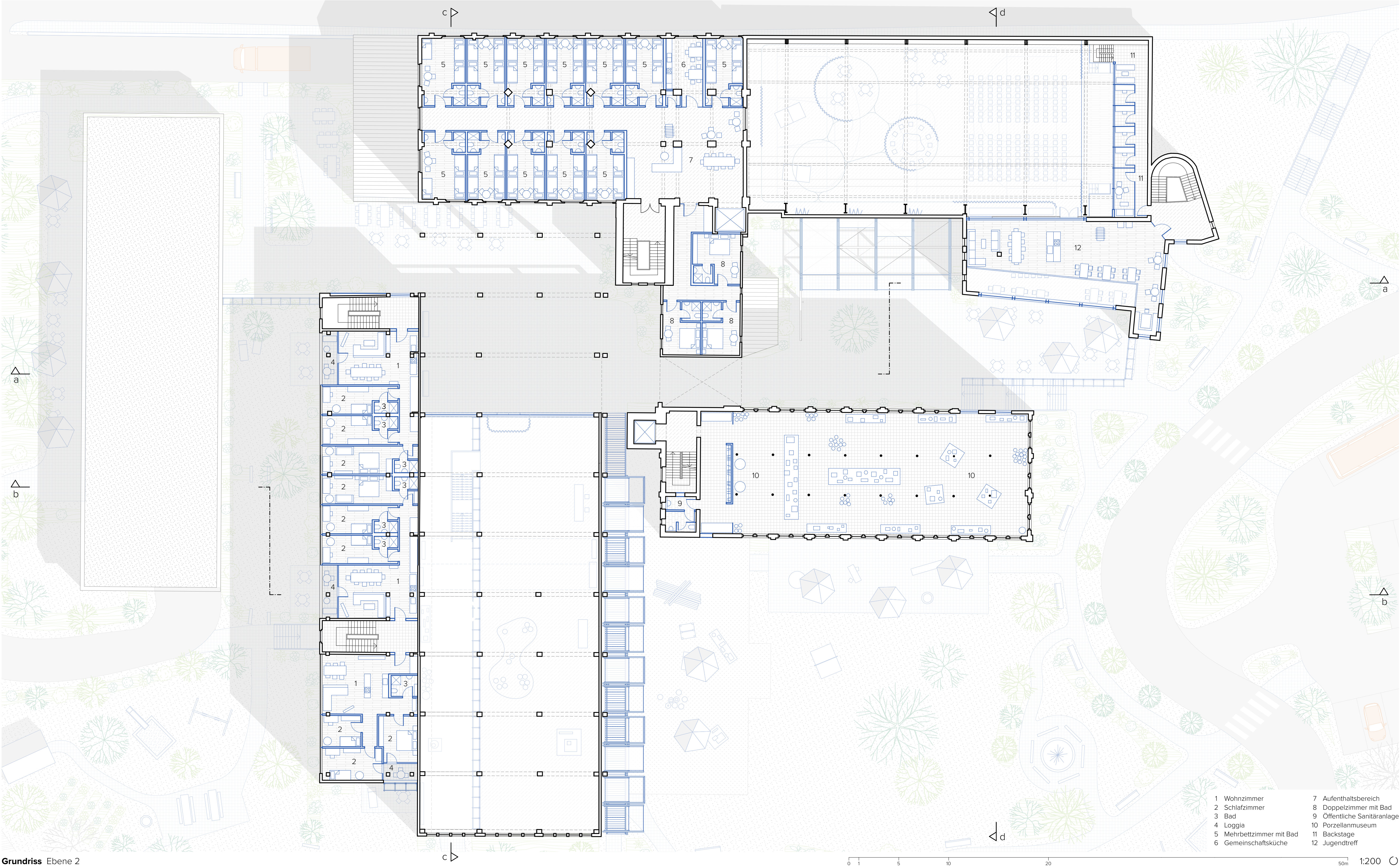
Grundriss Ebene 2
