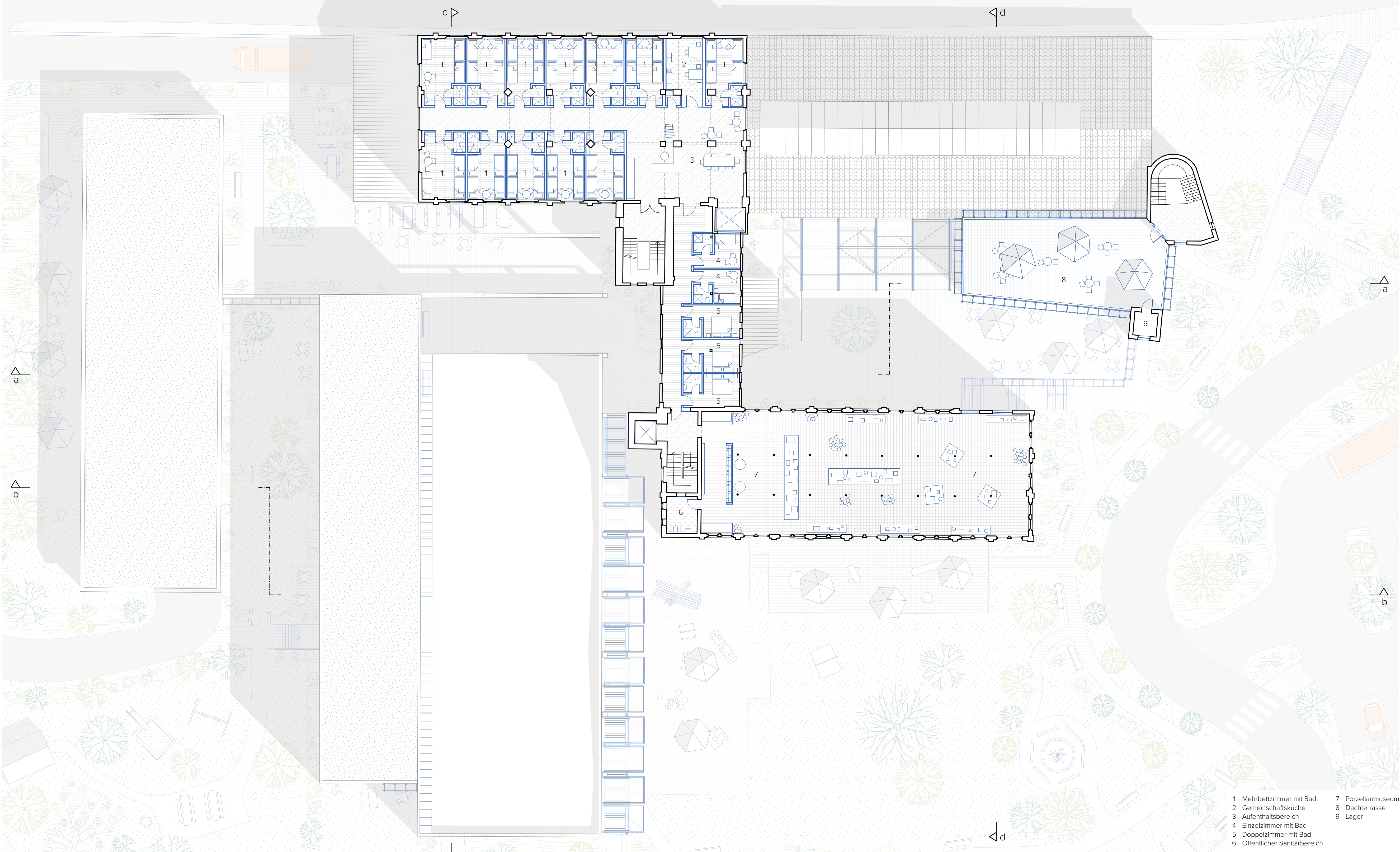
Grundriss Ebene 3
