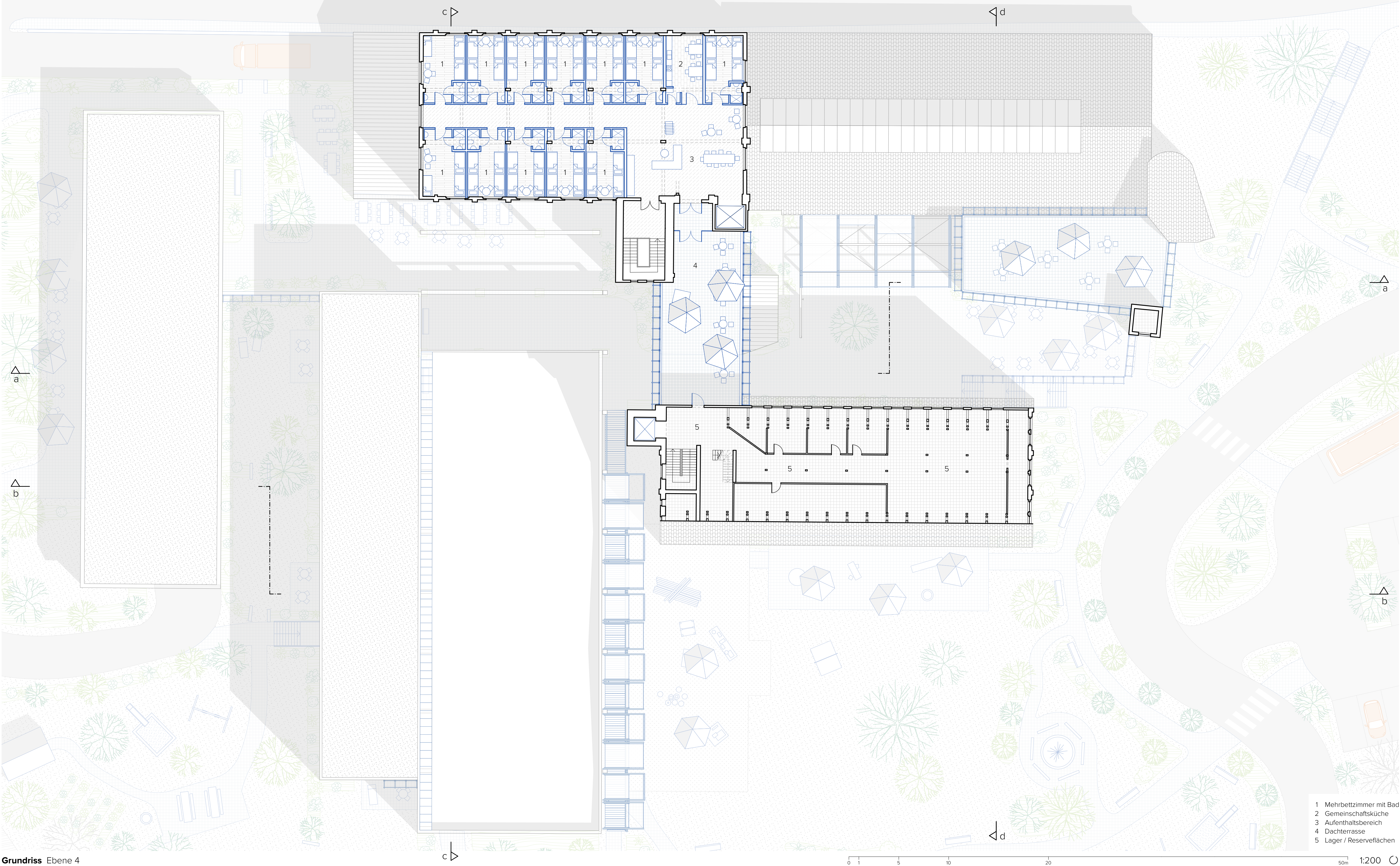
Grundriss Ebene 4
