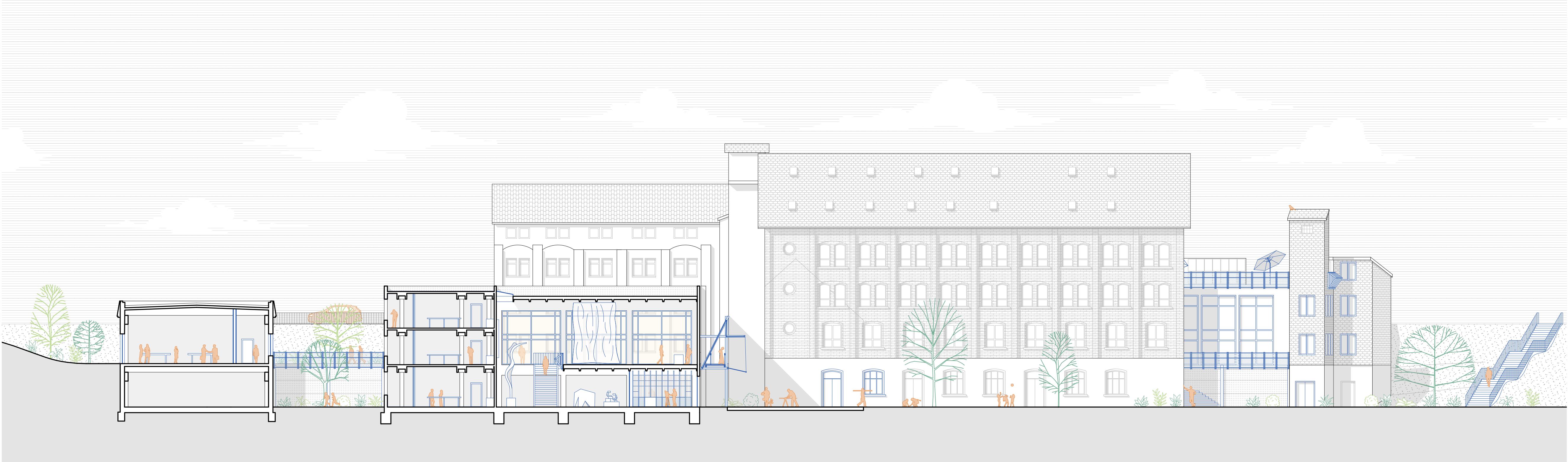
Querschnitt b-b Mensa, Weißlager vorne
