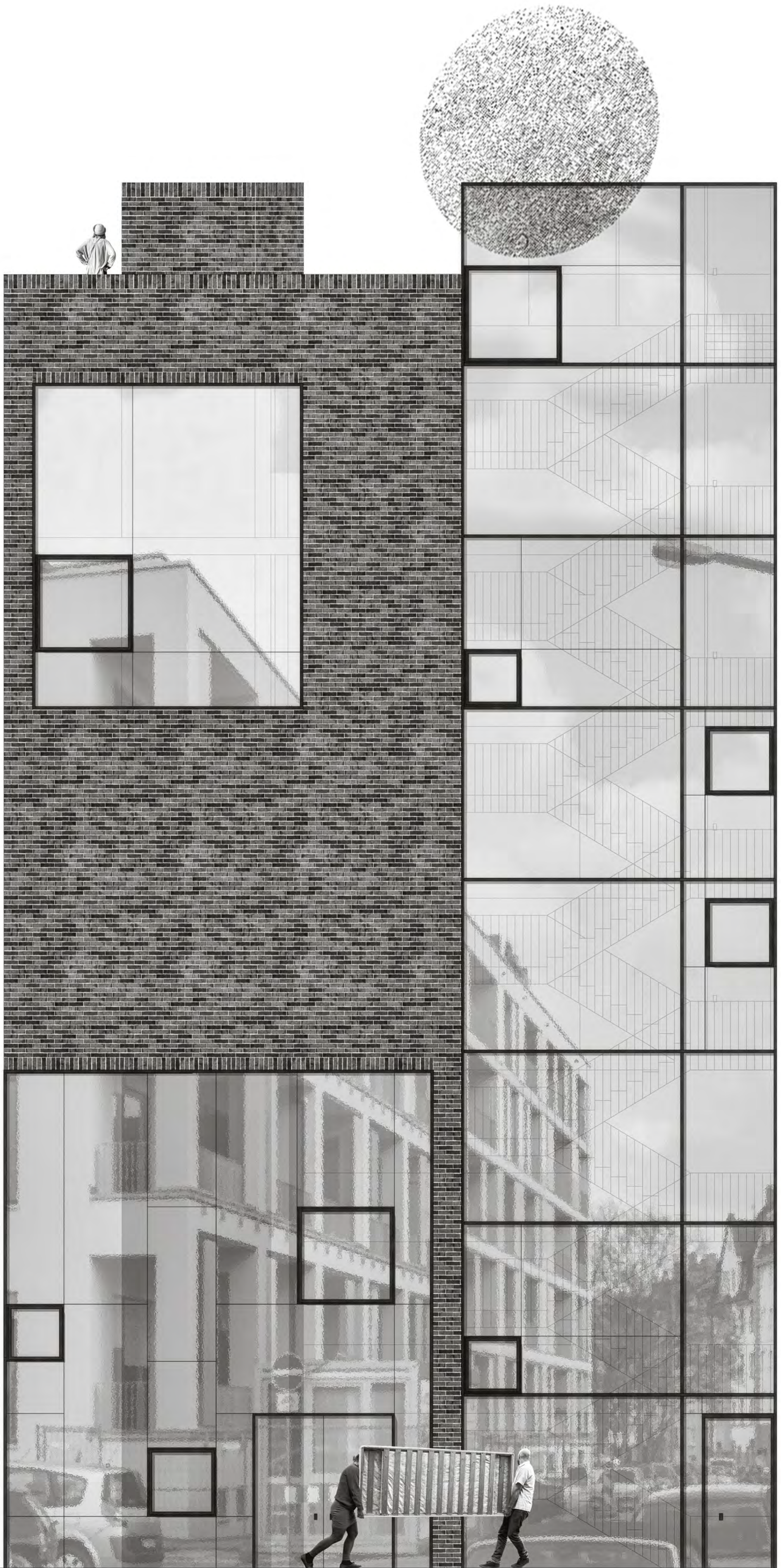
Fassadenchnitt M_1:50
