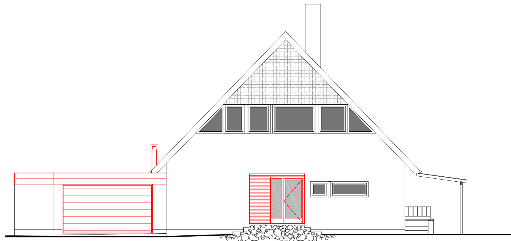
Ansicht Nord
