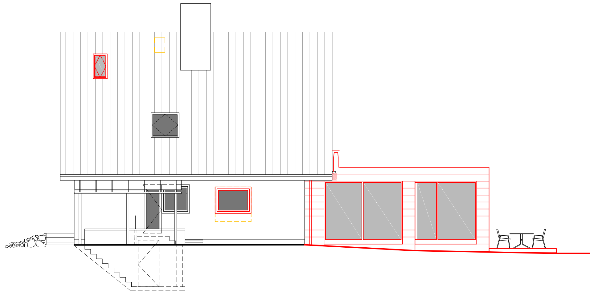
Ansicht West
