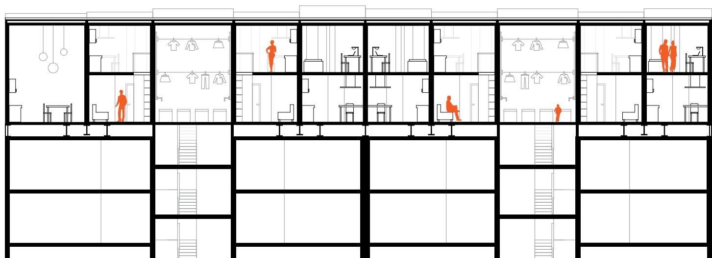
Schnitt C.C
