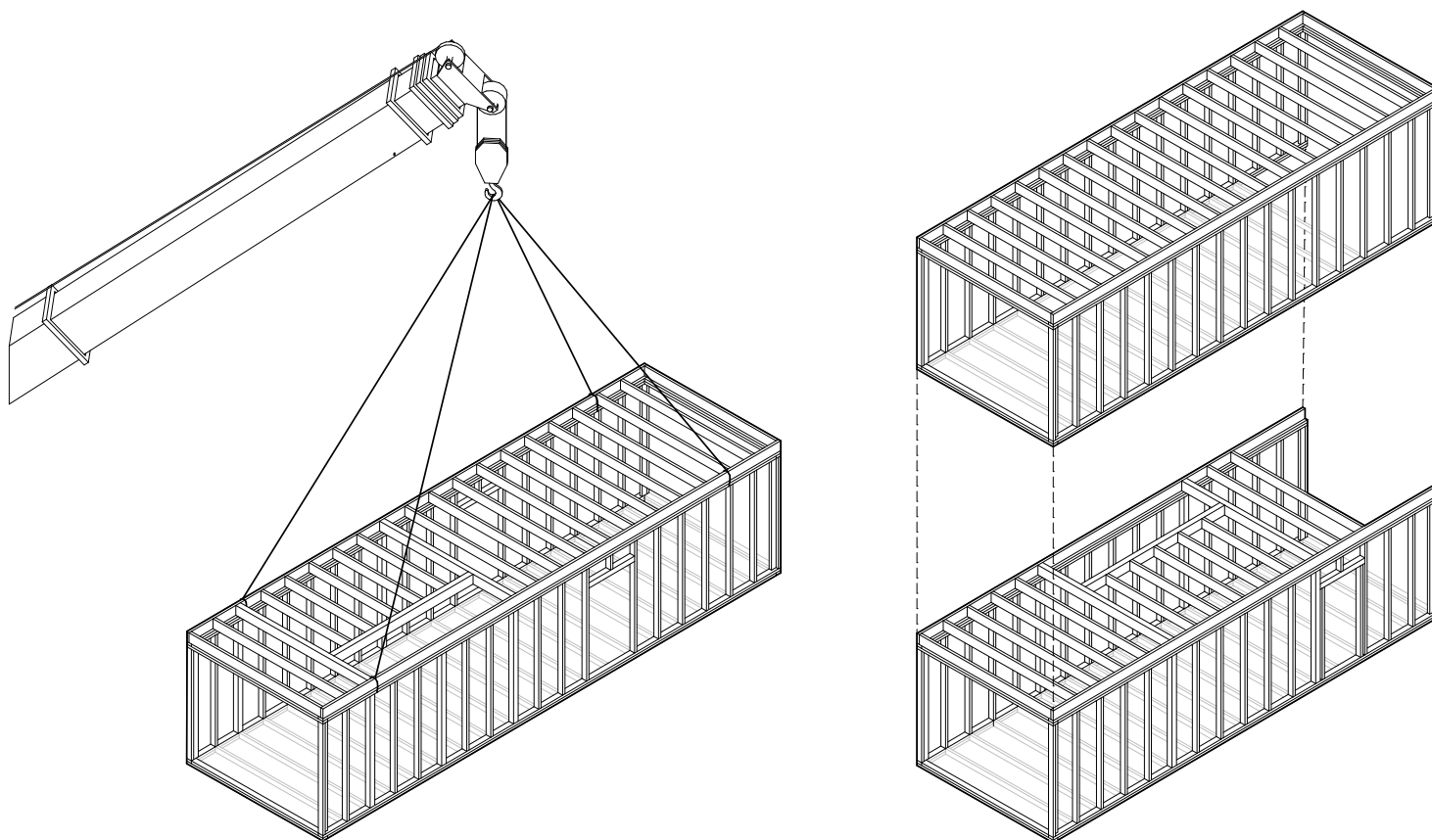
vorgefertigte Raumzellen in Holzrahmenbauweise
