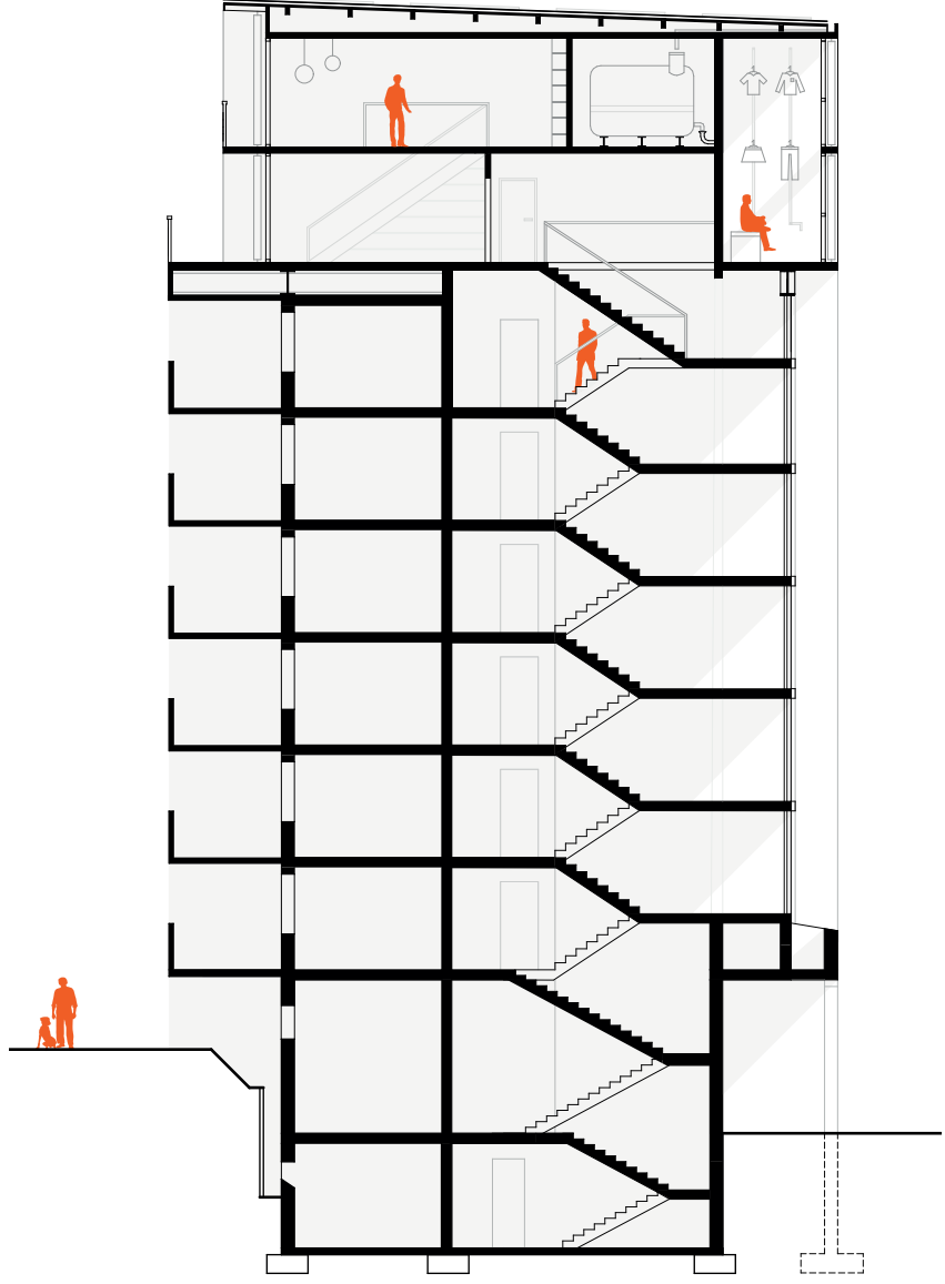
Schnitt B.B
