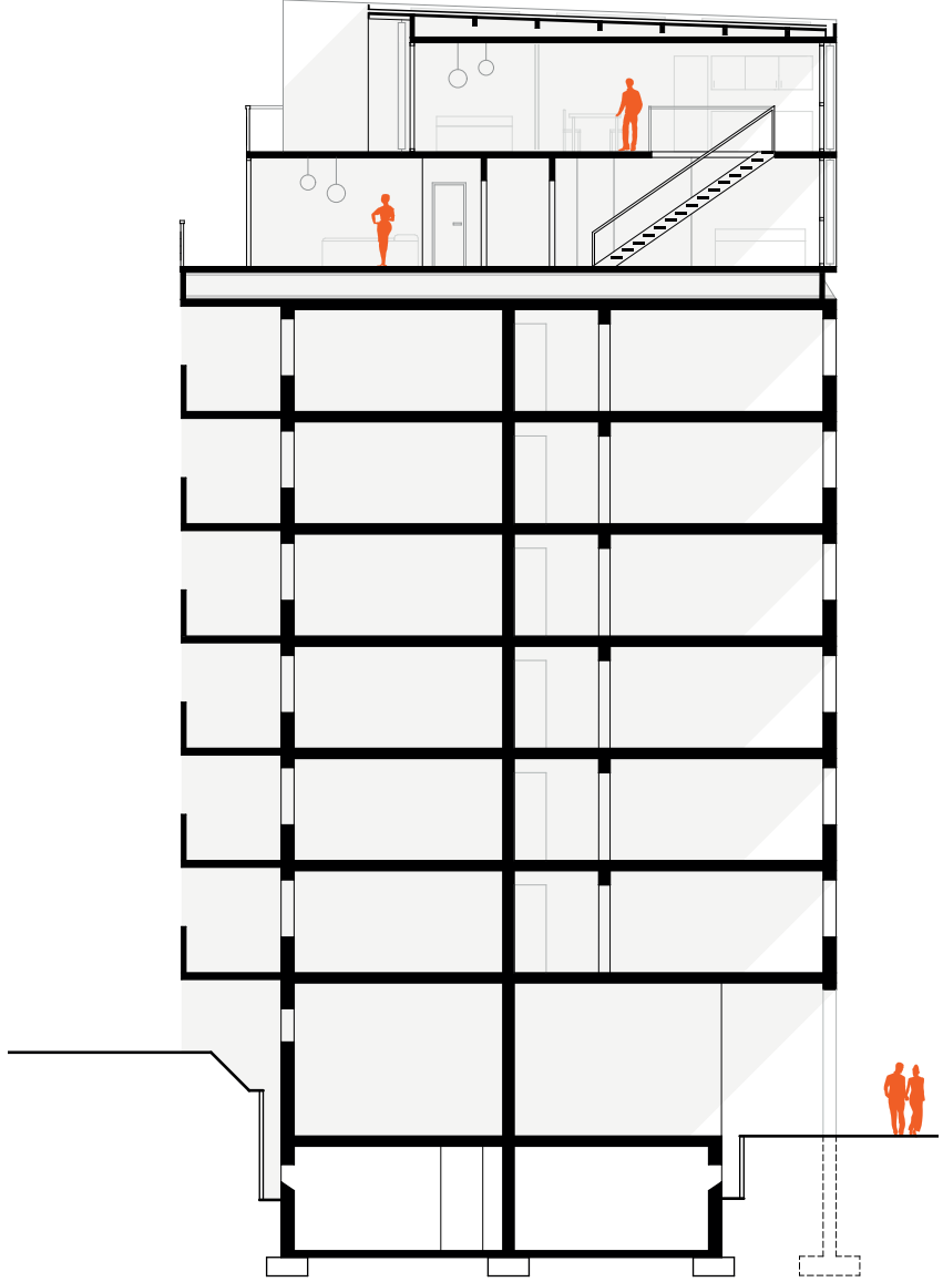
Schnitt A.A
