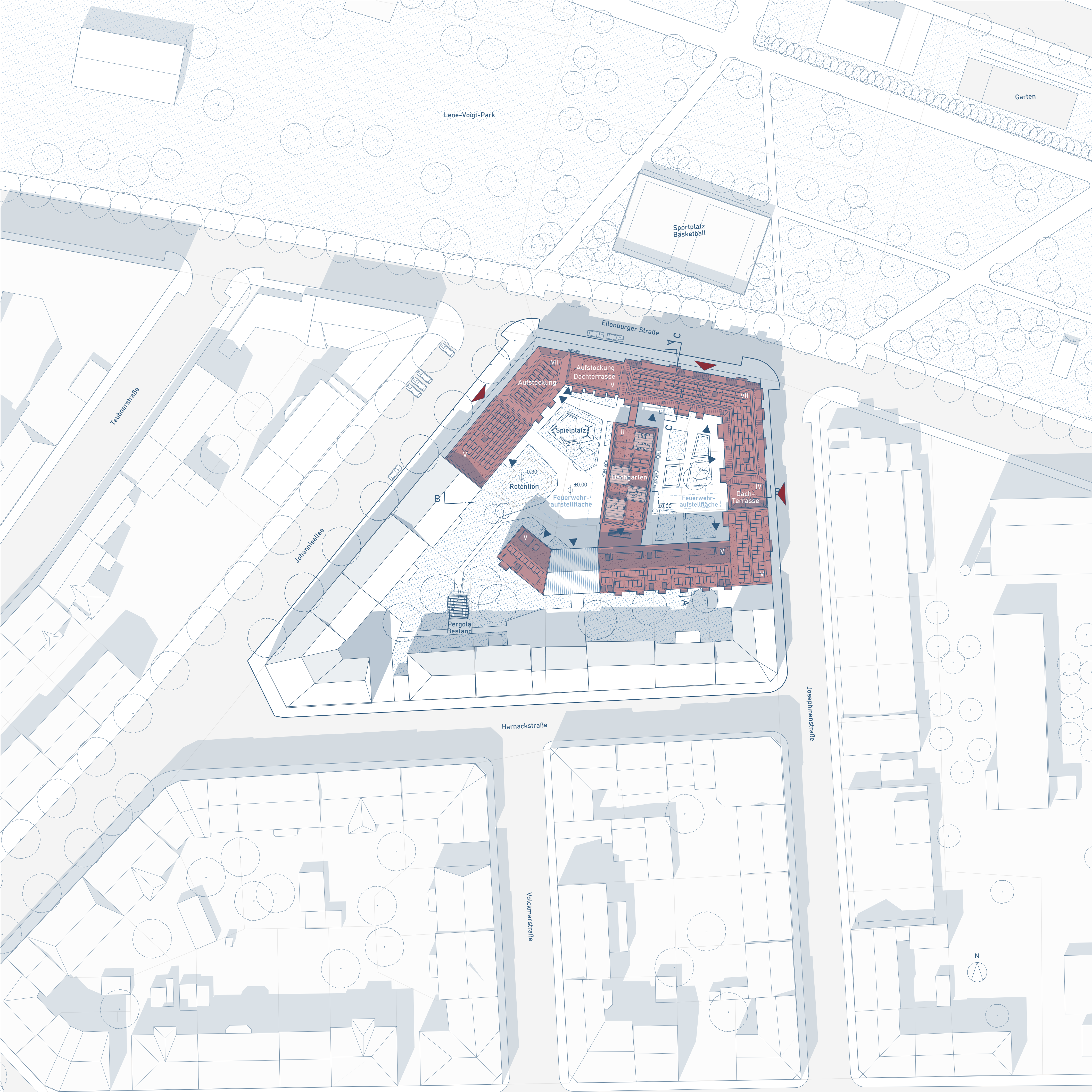
LAGEPLAN
