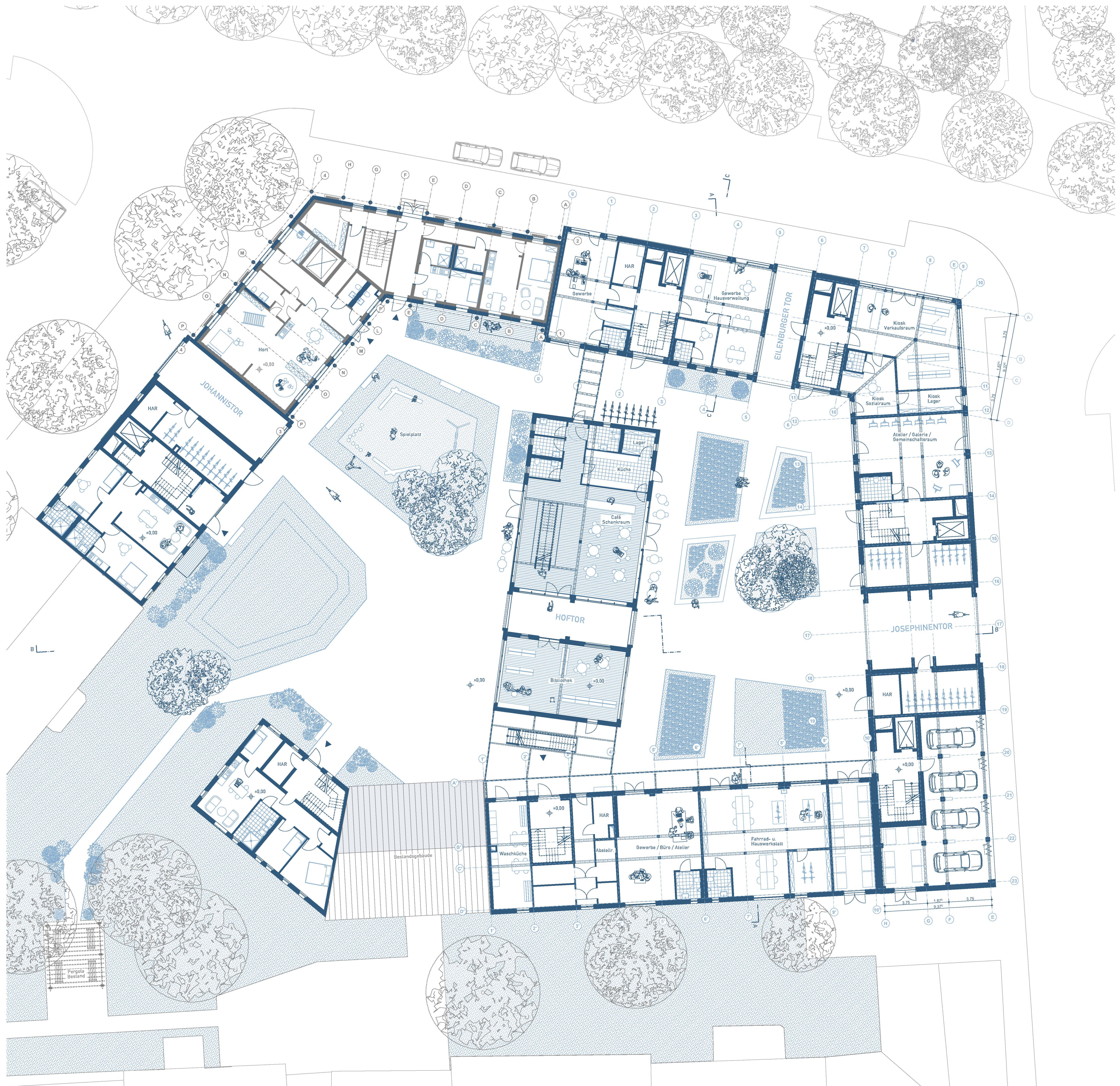
GRUNDRISS EG
