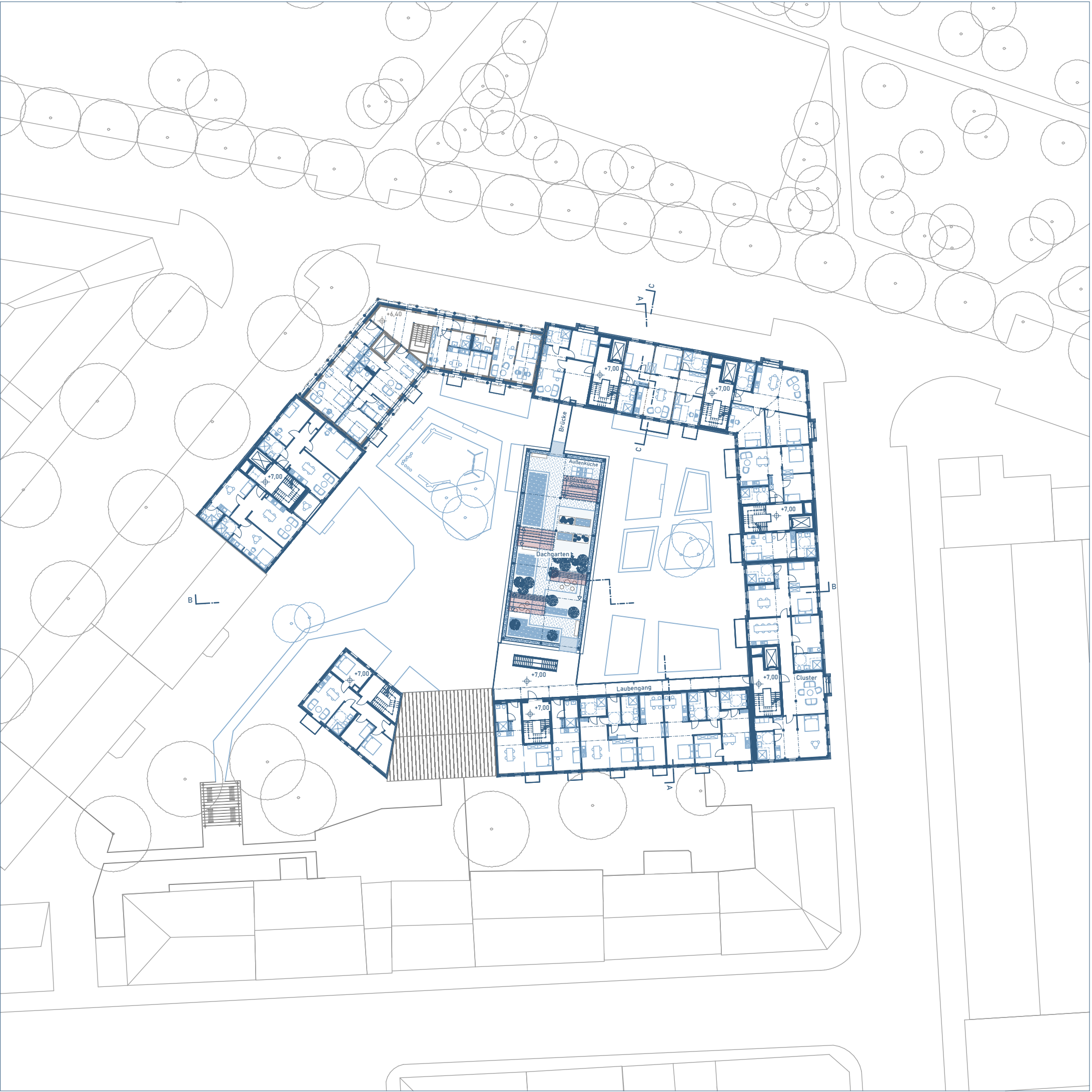
GRUNDRISS 2. OG
