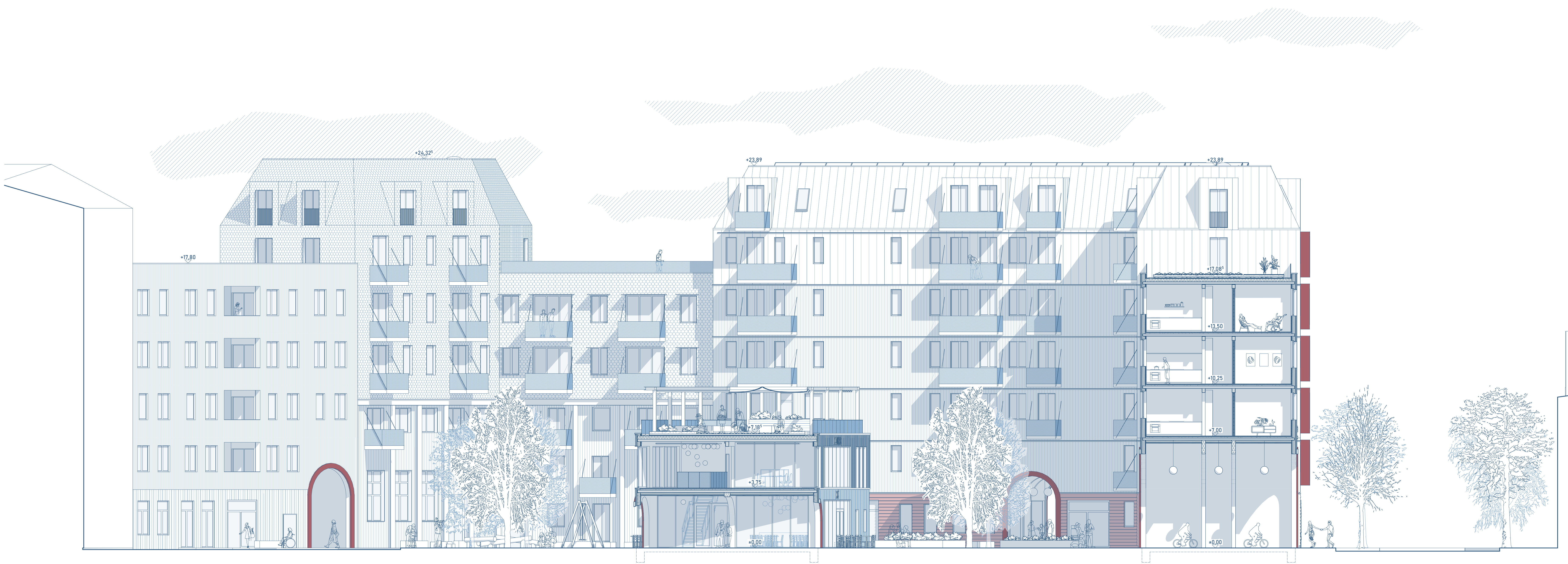
Schnitt B-B
