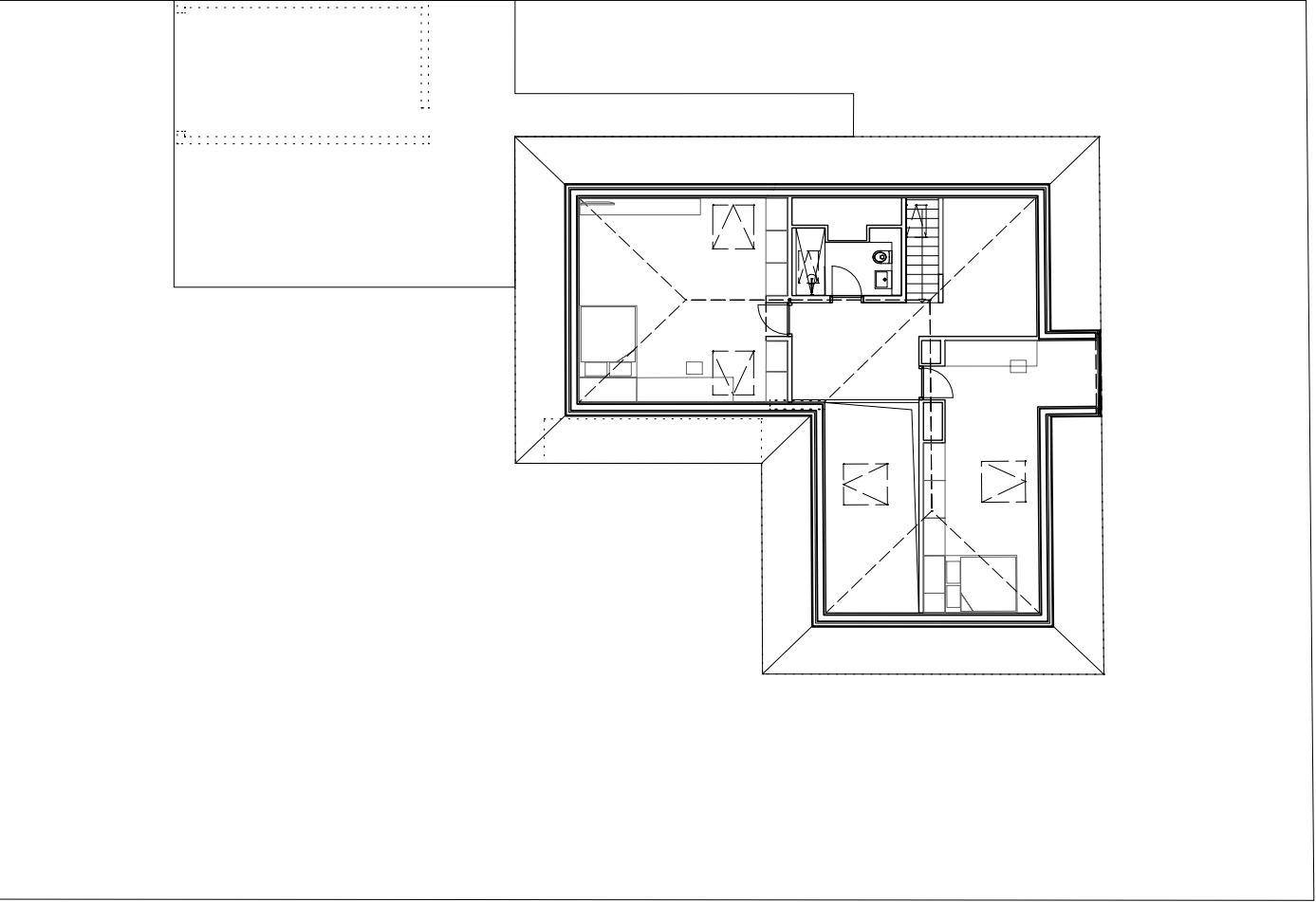
GRUNDRISS DG
