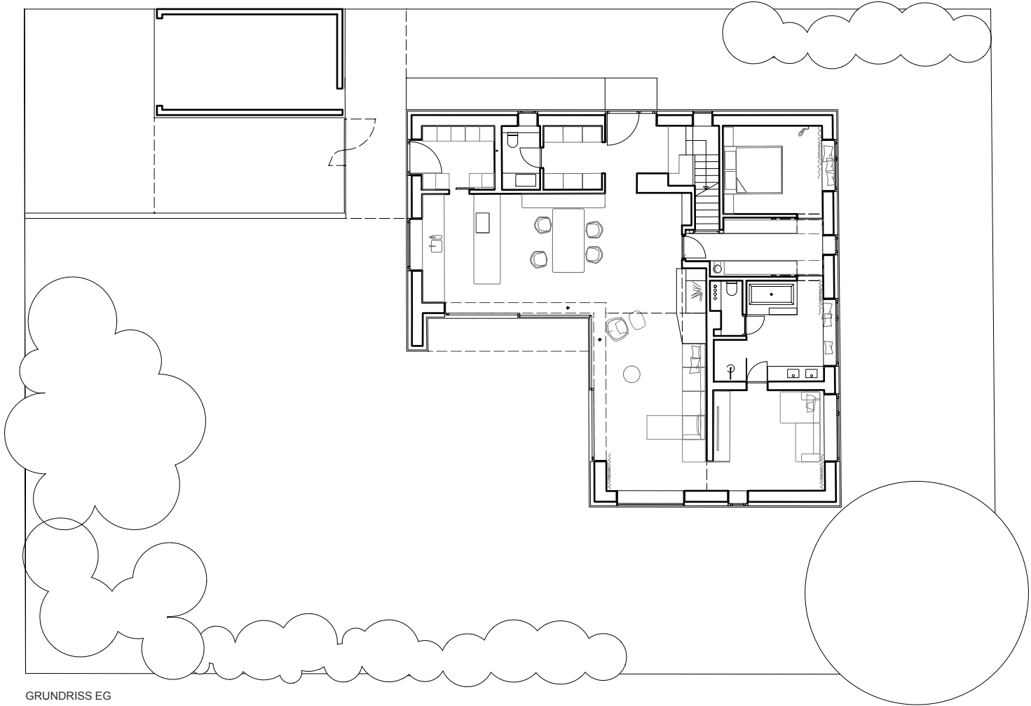
GRUNDRISS EG
