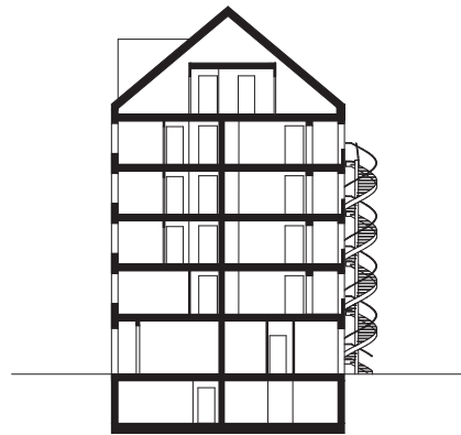
Schloßstrasse, Frankfurt am Main - Schnitt
