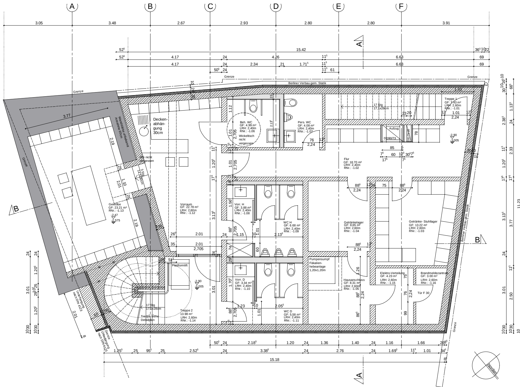
BV 050.Weinkulturhaus Bürgstadt - M 1:50 - UG (Ausschnitt)
