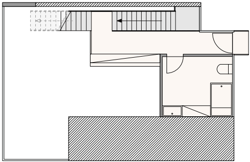
3. Obergeschoss
