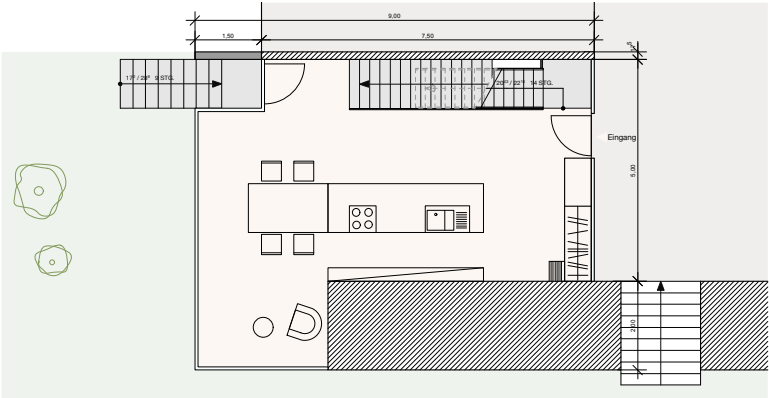
Erdgeschoss
