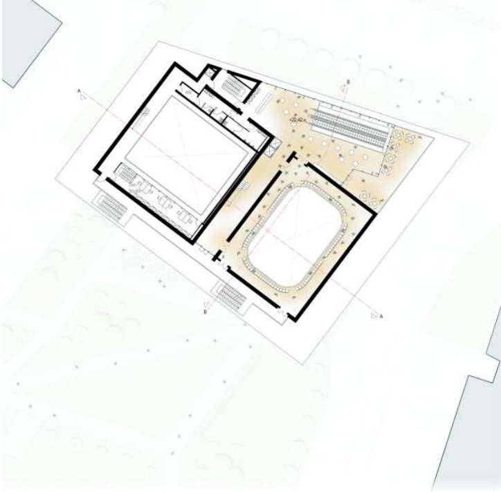
5. Obergeschoss, Vision 1 M 1:200
