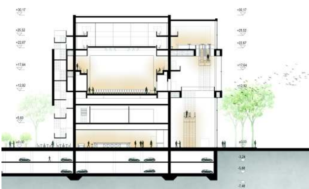
Querschnitt B-B, Vision 1 M 1:200
