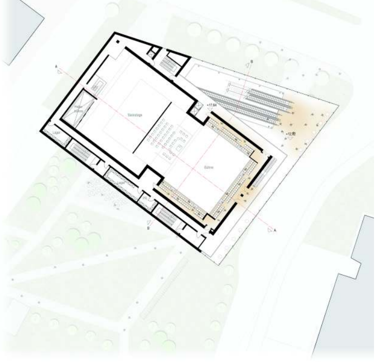
5. Obergeschoss, Vision 2 M 1:200
