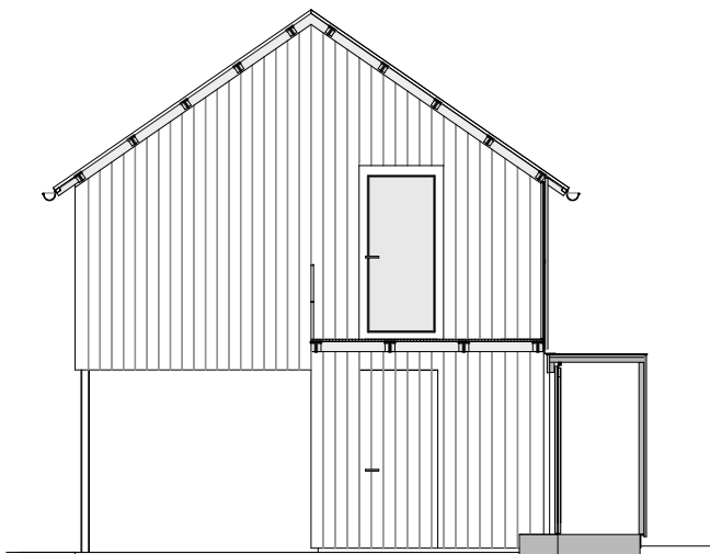
SCHNITT B-B
