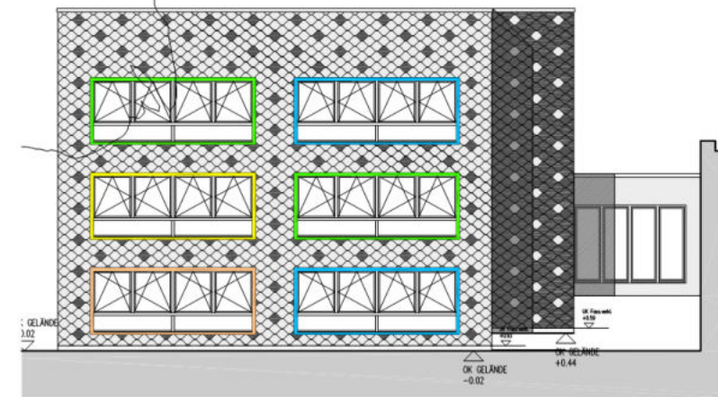
Ansicht Süd
