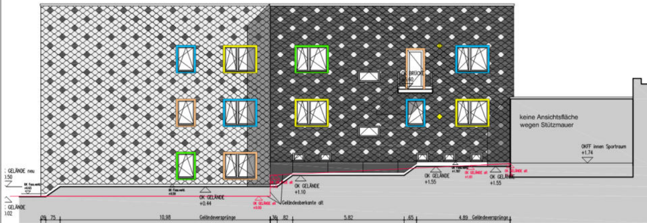
Ansicht Ost
