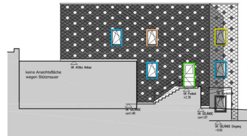
Ansicht Nord
