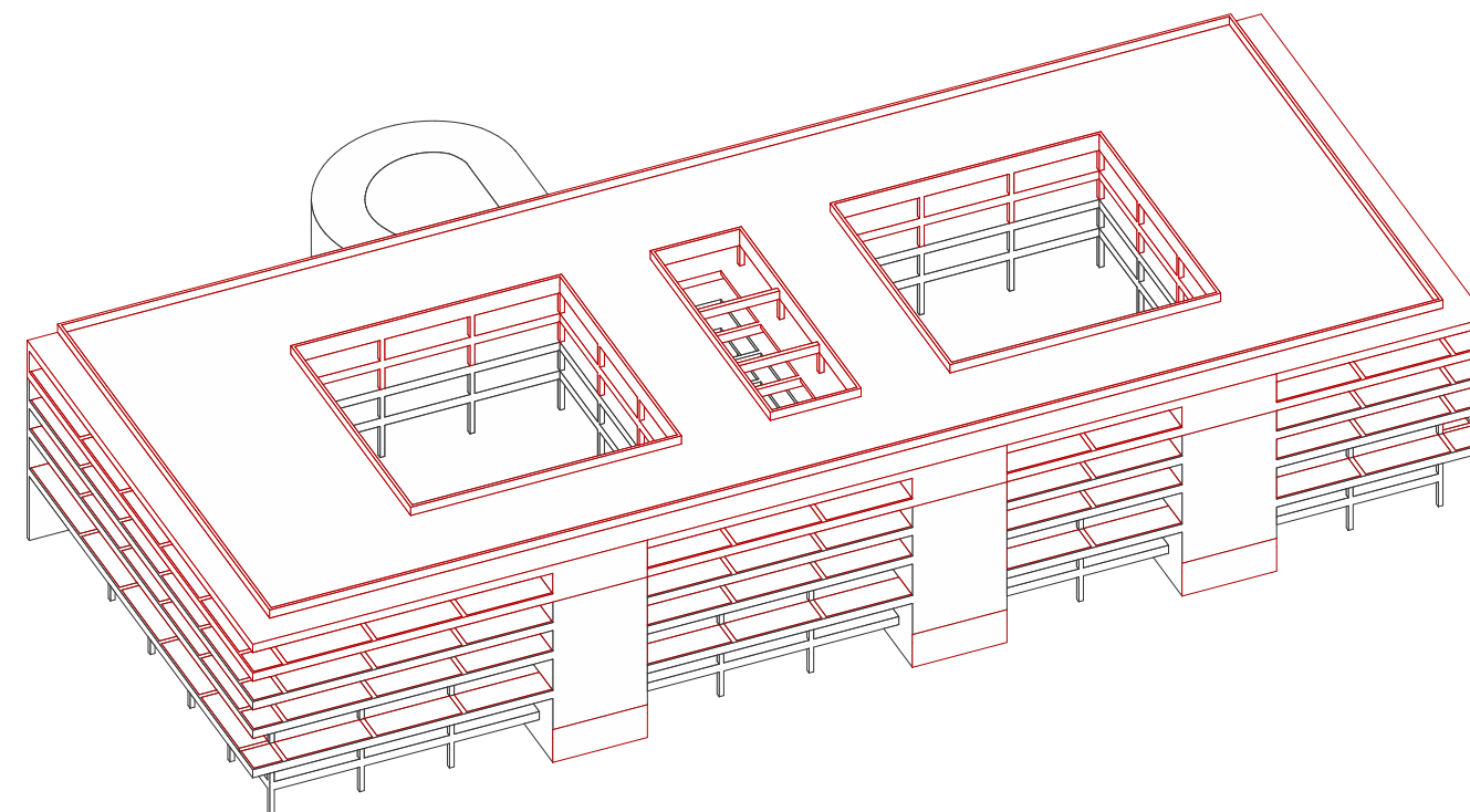
Tragstruktur Neu
