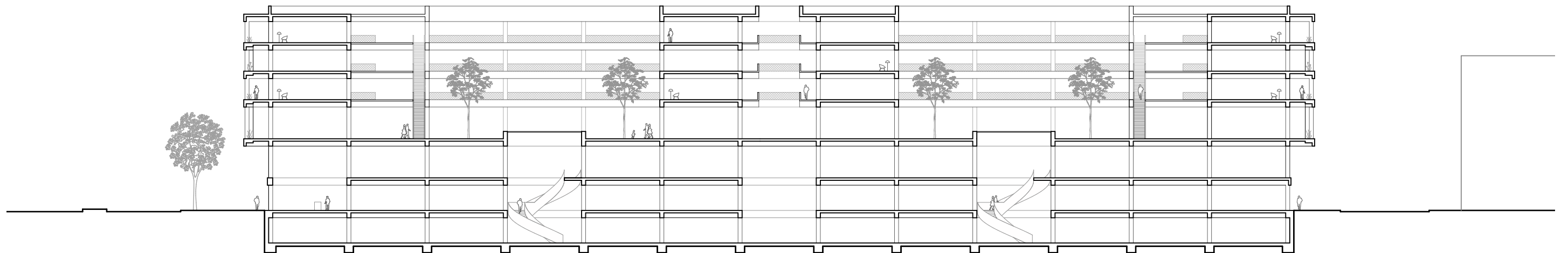
Längsschnitt
