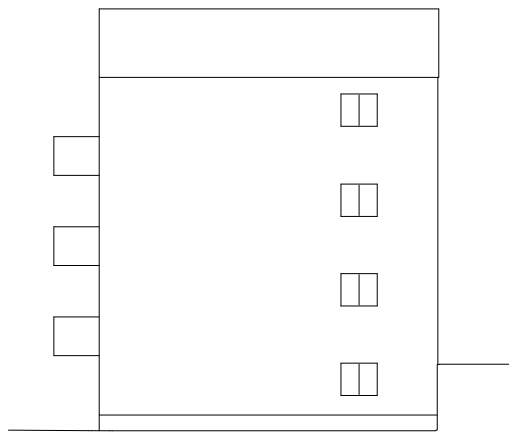
0 1 3 5 10 ANSICHT SÜD
