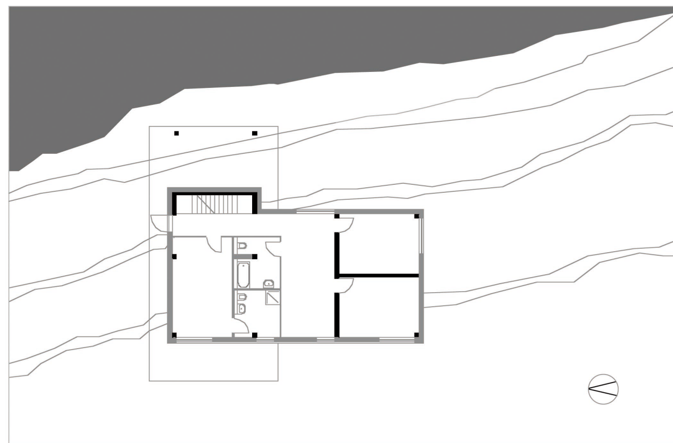
Ebene 1 Individualräume
