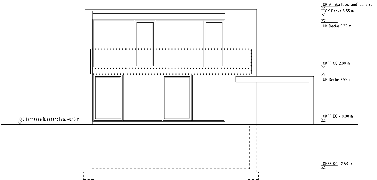
Ansicht Süd
