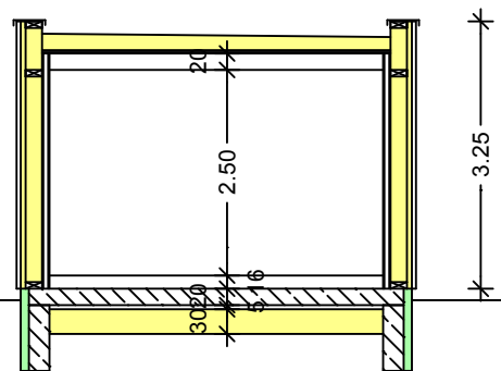
Systemschnitt Anbau
