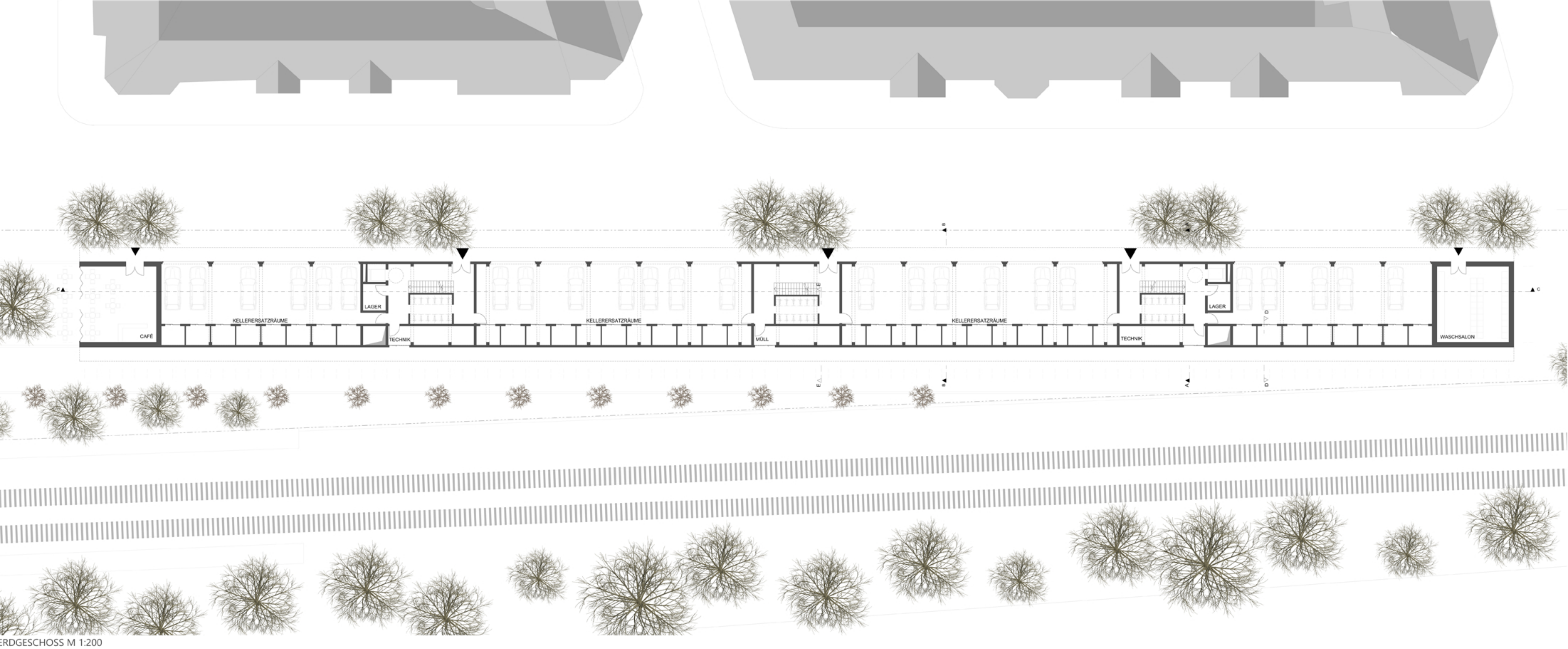
ERDGESCHOSS M 1:200
