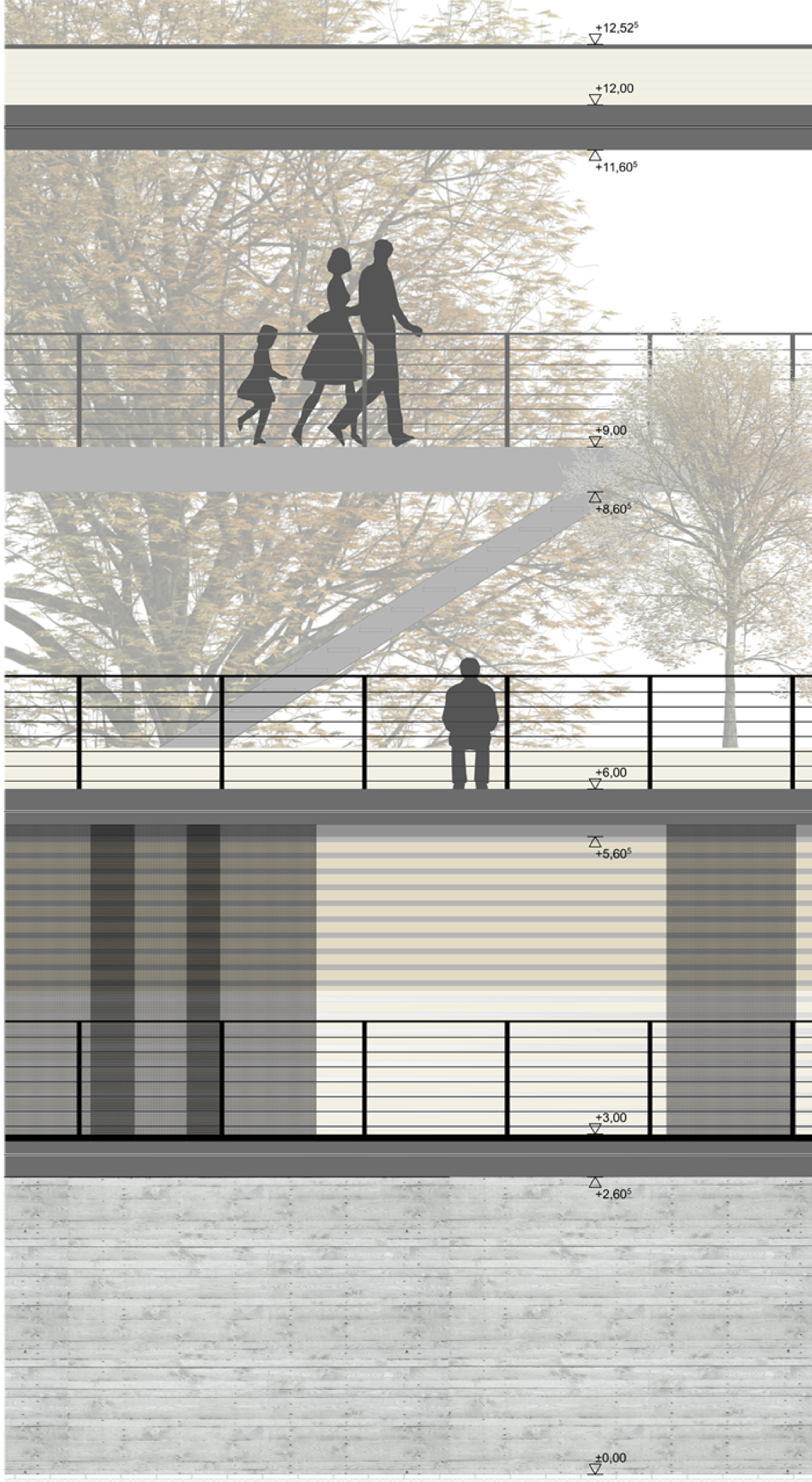
TEILANSICHT M 1:20
