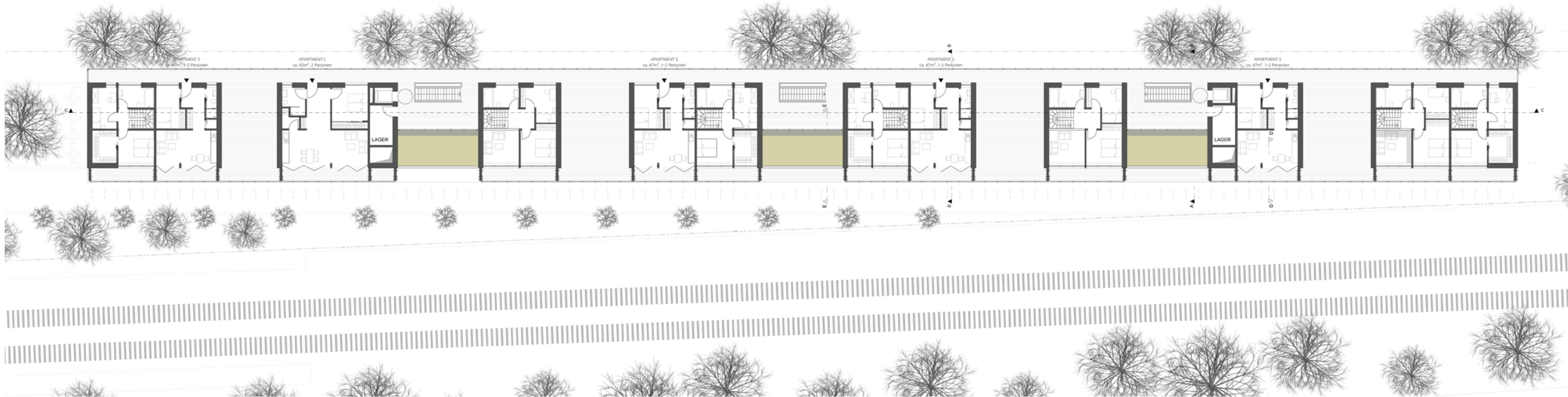
3. OBERGESCHOSS M 1:200
