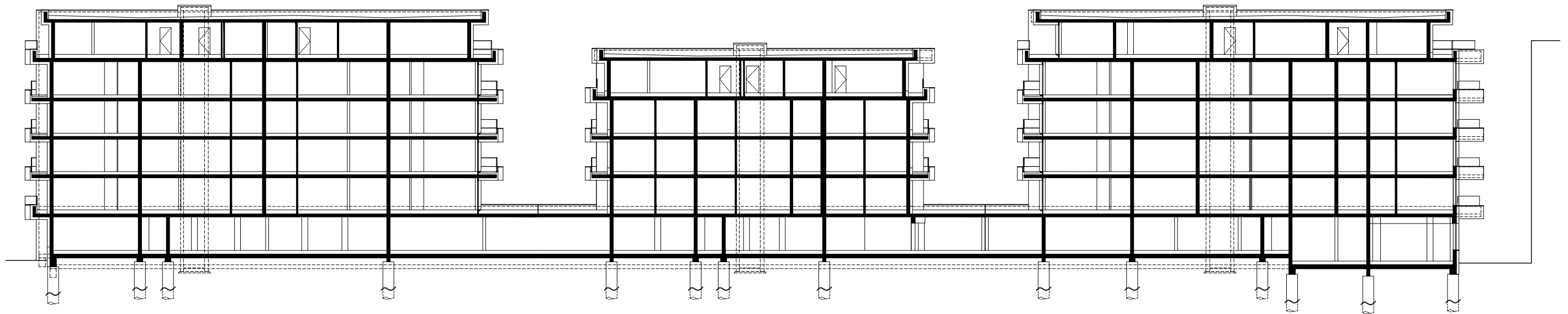
Längsschnitt
