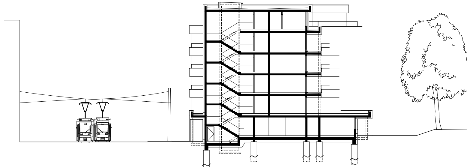
Querschnitt
