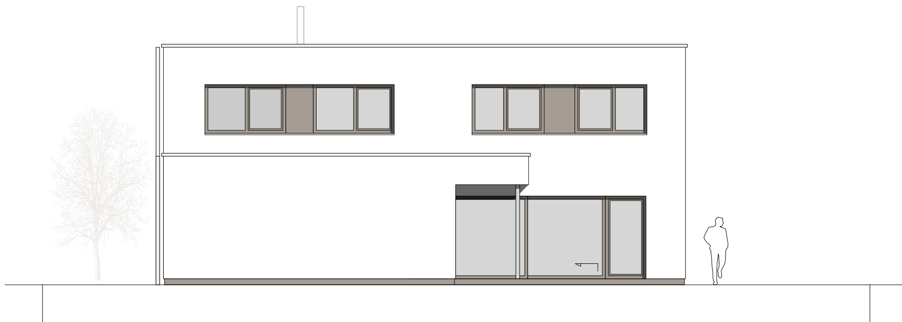
Ansicht West
