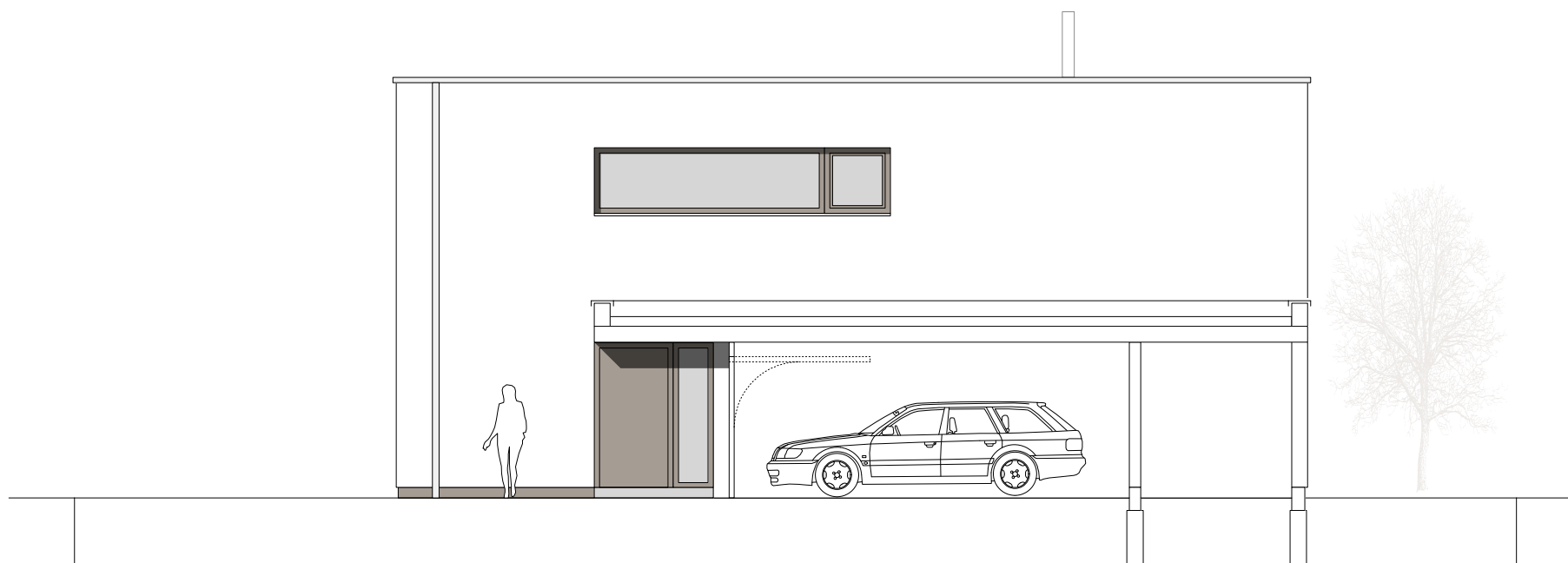
Ansicht Ost
