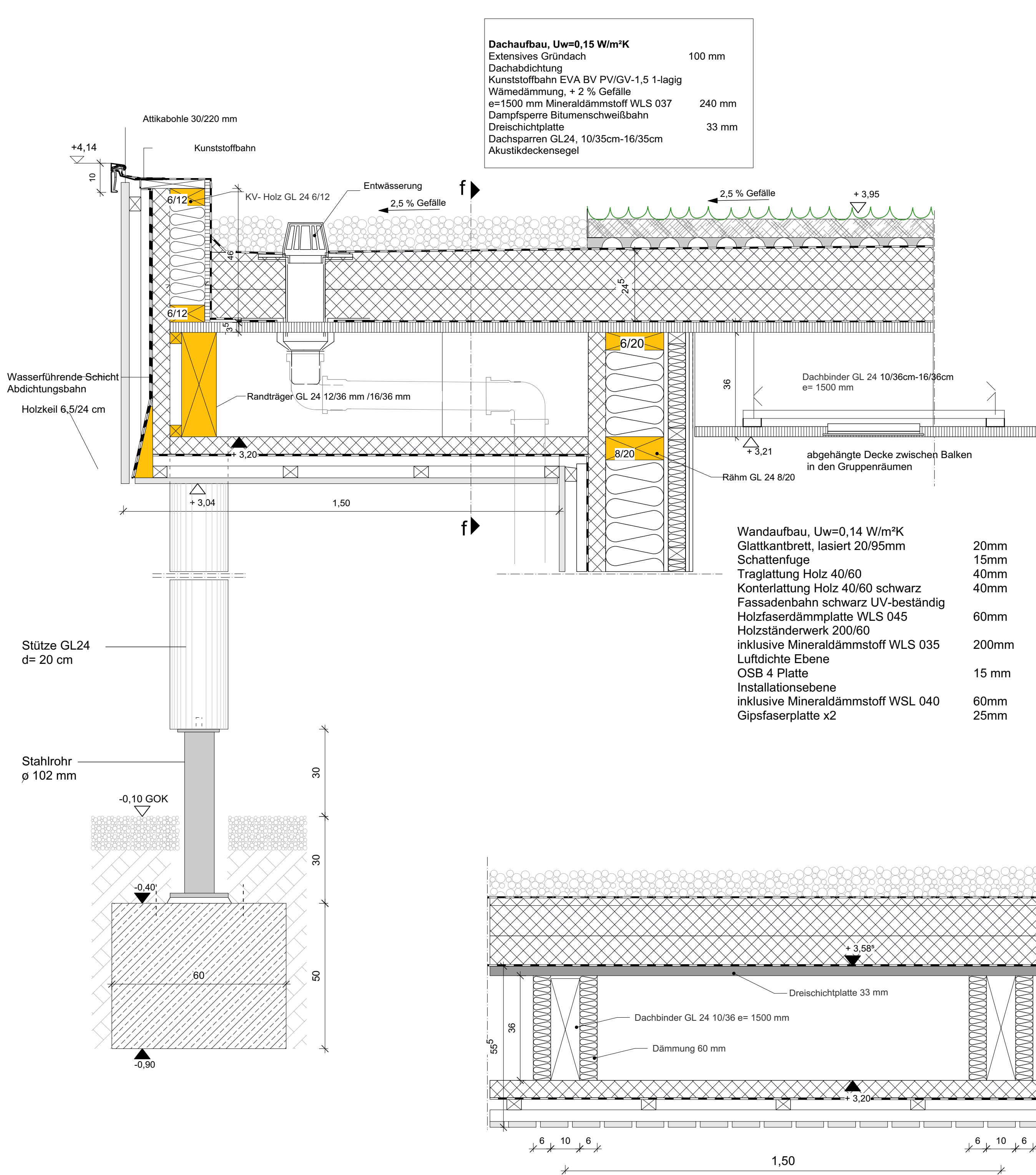
Schnitt f-f
