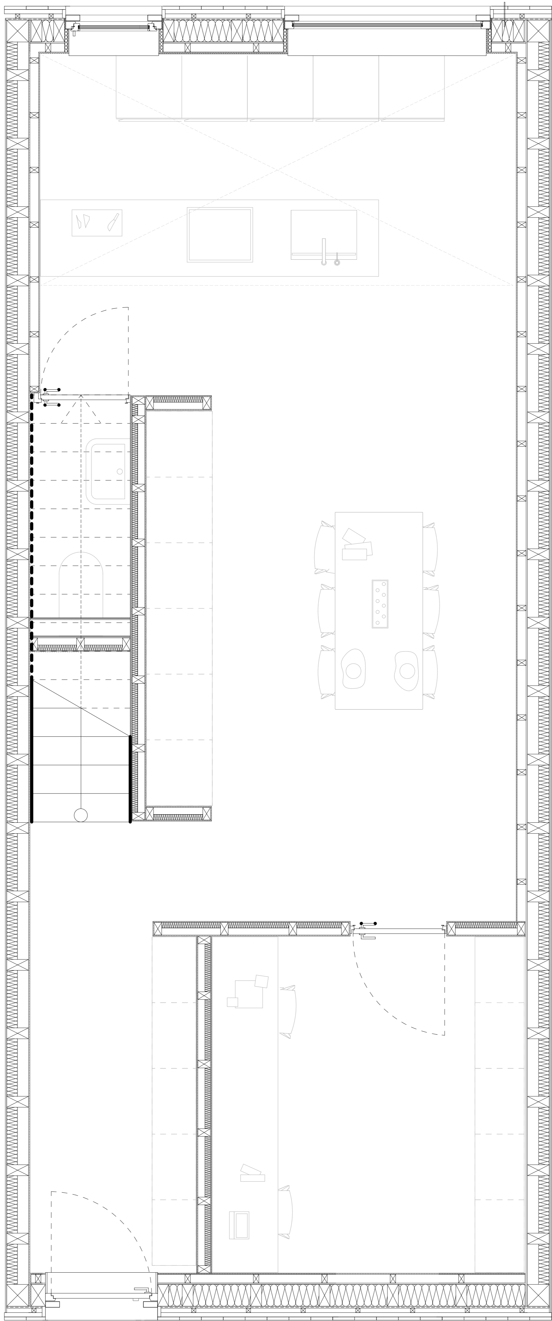
Grundriss Erdgeschoss M1:50
