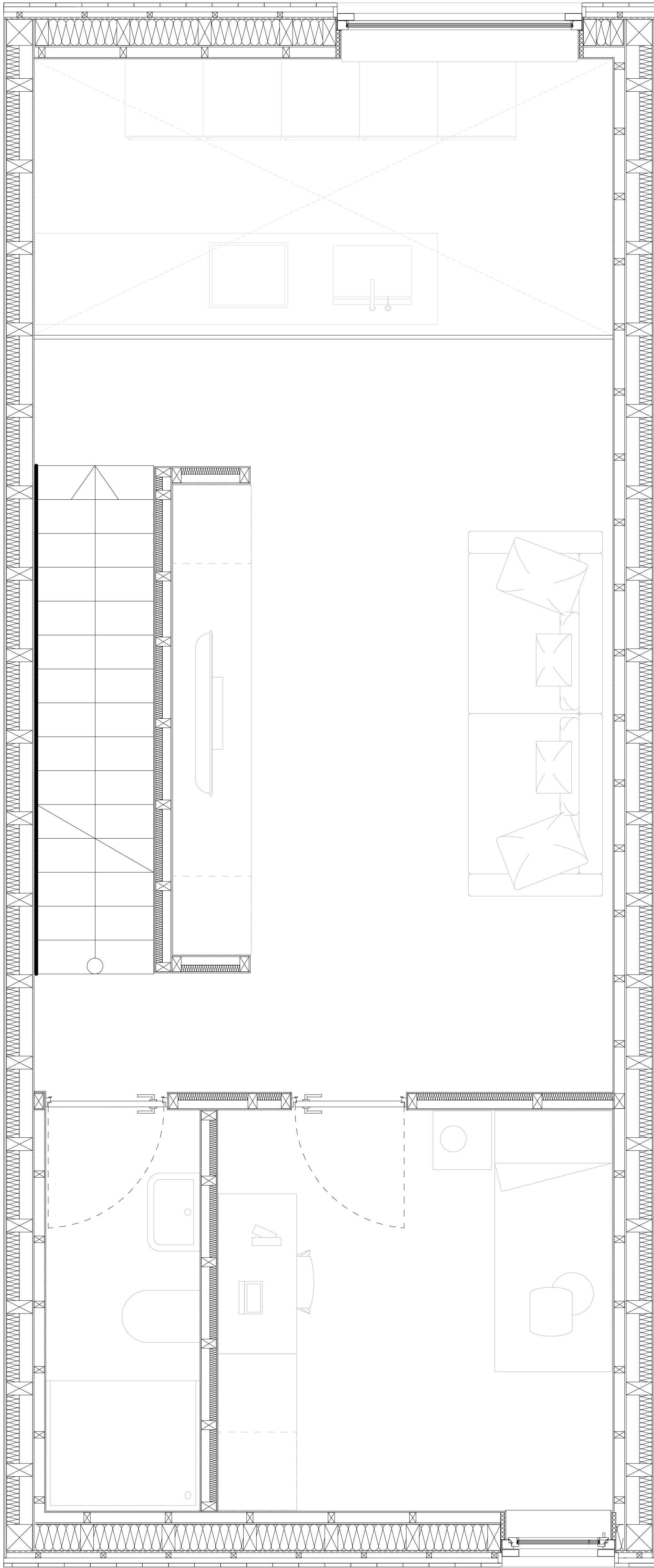
Grundriss 1. Obergeschoss M1:50
