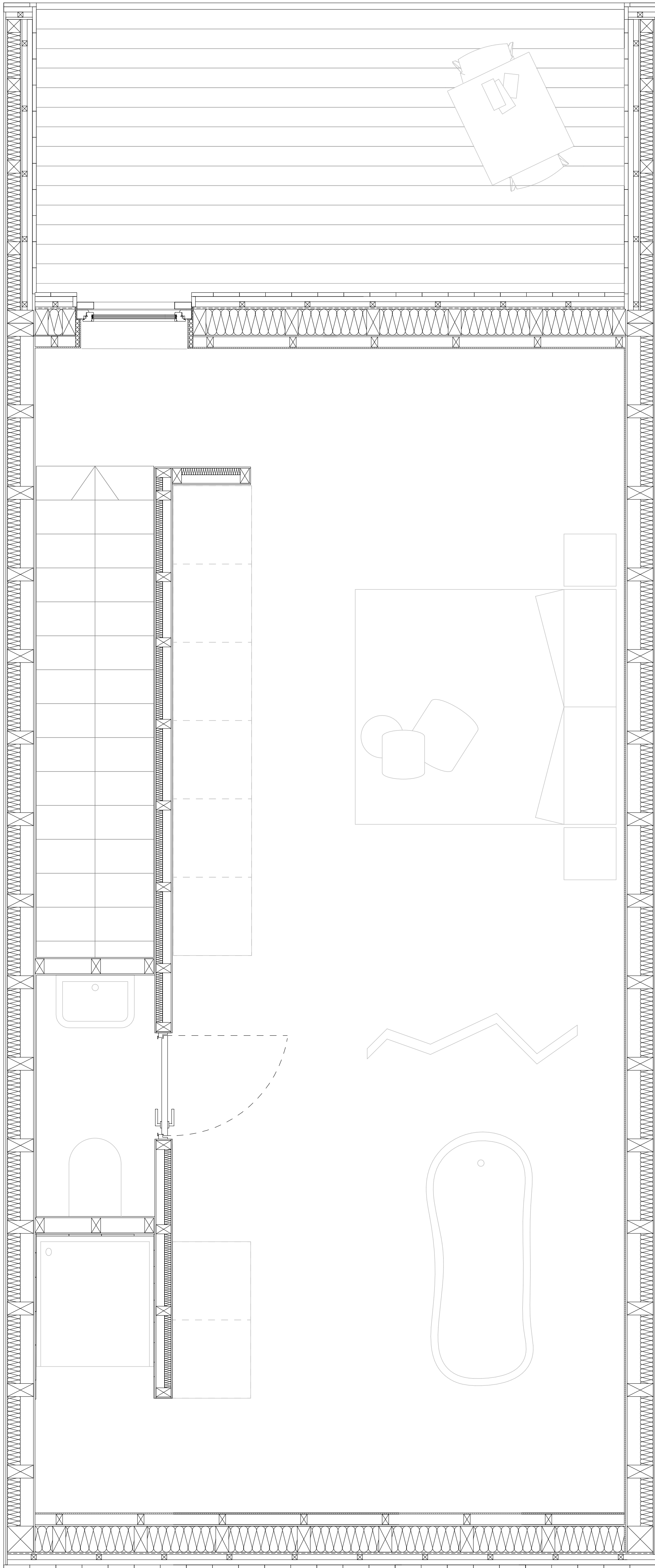
Grundriss 2. Obergeschoss M1:50
