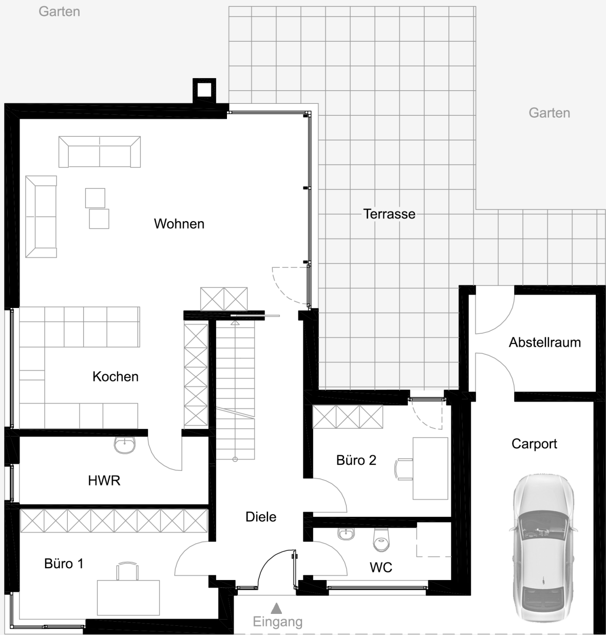
Grundriss Erdgeschoss
