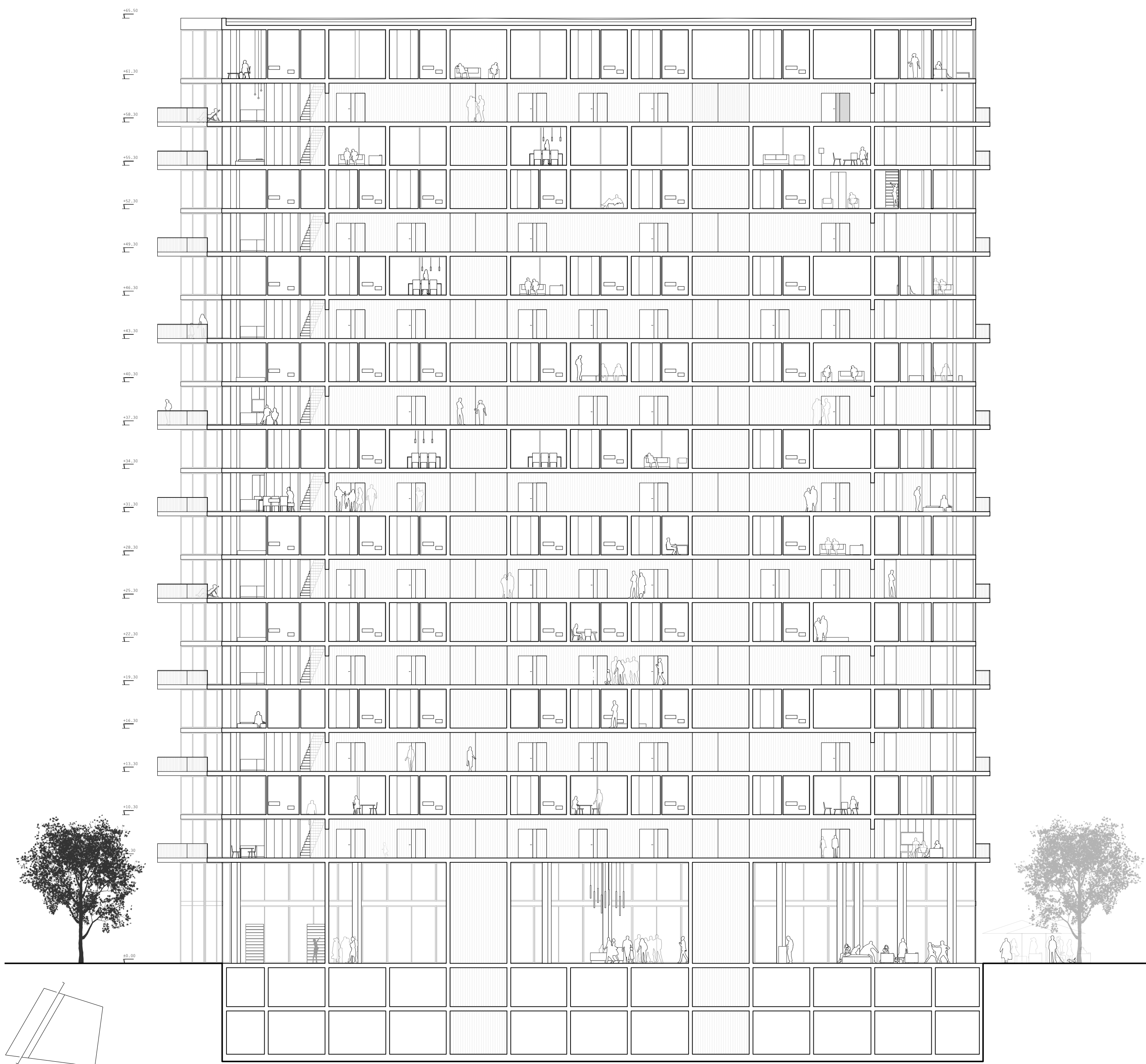
Schnitt 01 1.200
