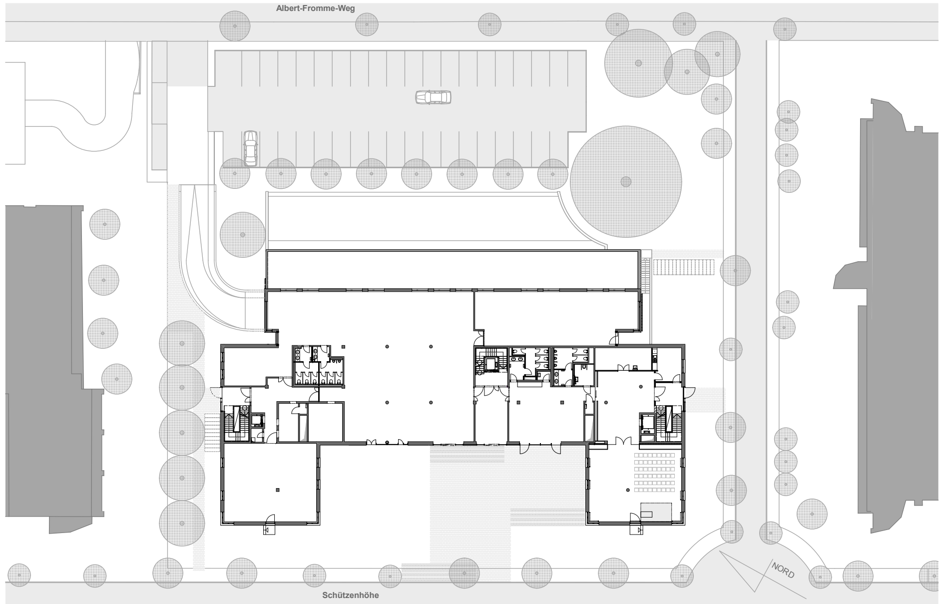
Grundriss Erdgeschoss | M 1:500
