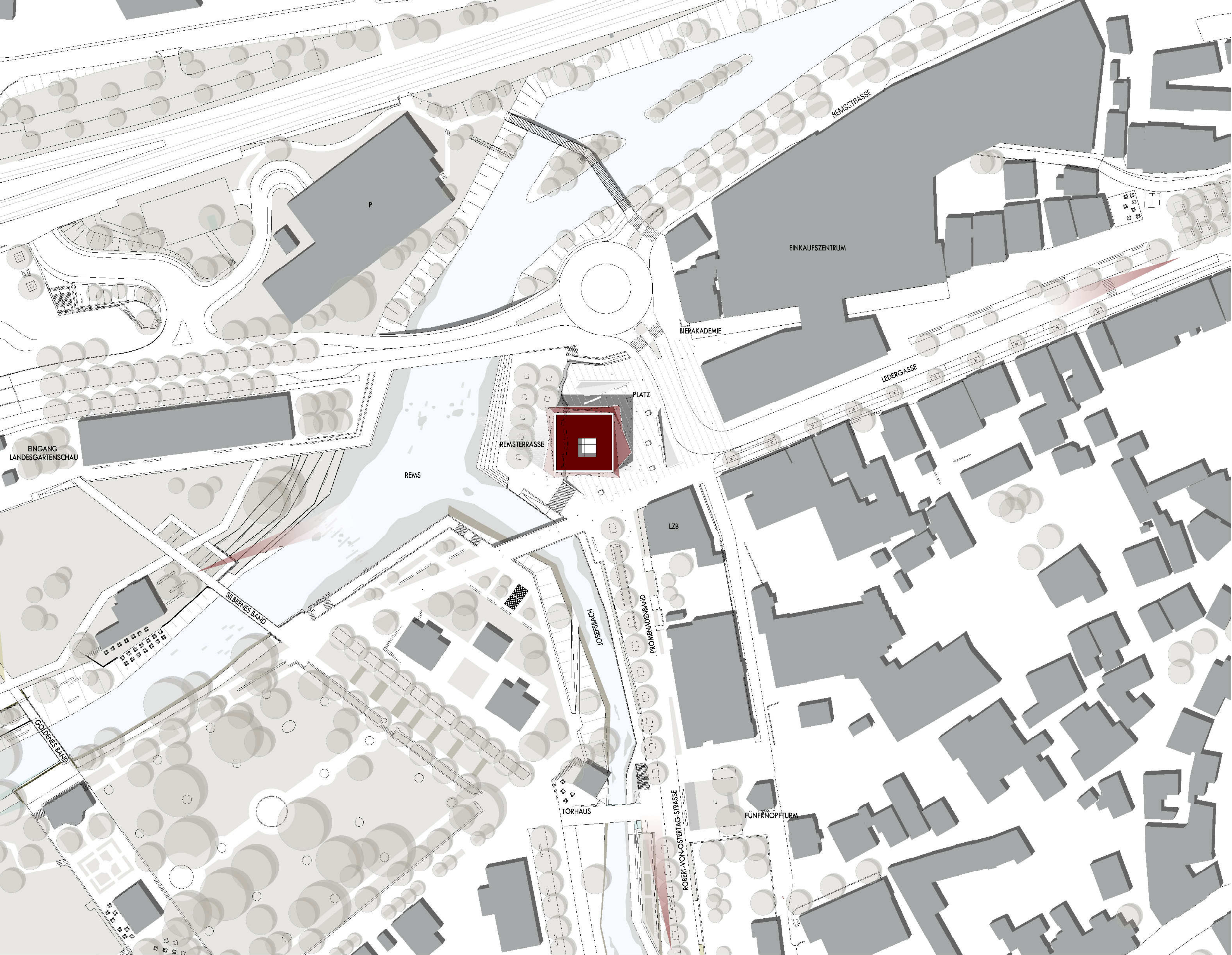
LAGEPLAN M 1.500
