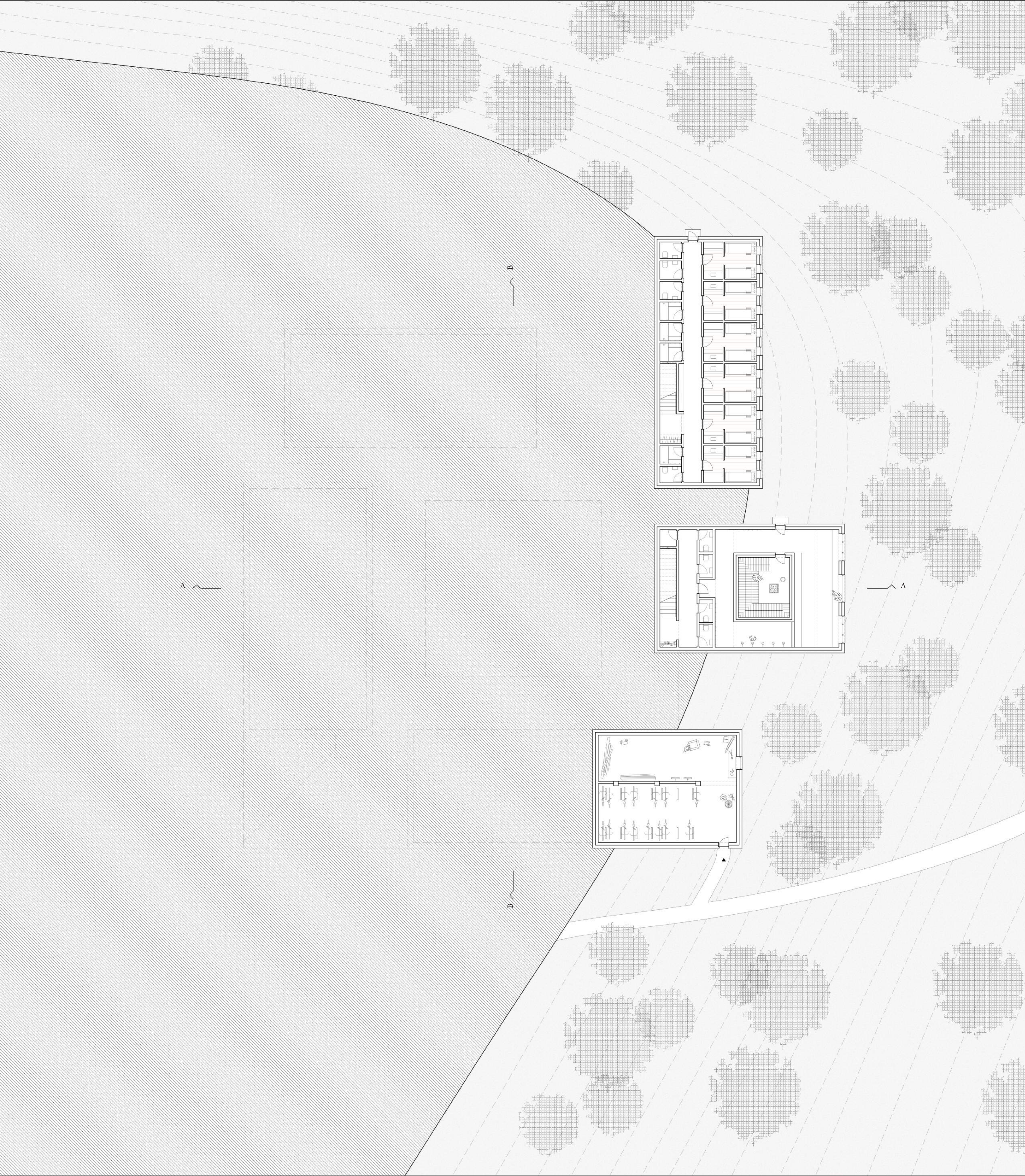
Grundriss Untergeschoss
